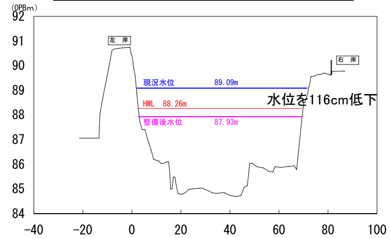
黒津地点(大戸川 約1km付近)横断面図
