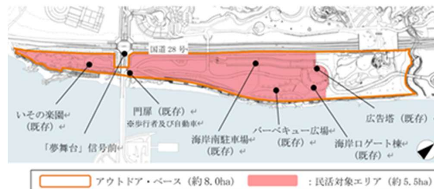
海岸ゾーン「アウトドア・ベース」(民活対象：約5.5ha)平面図
