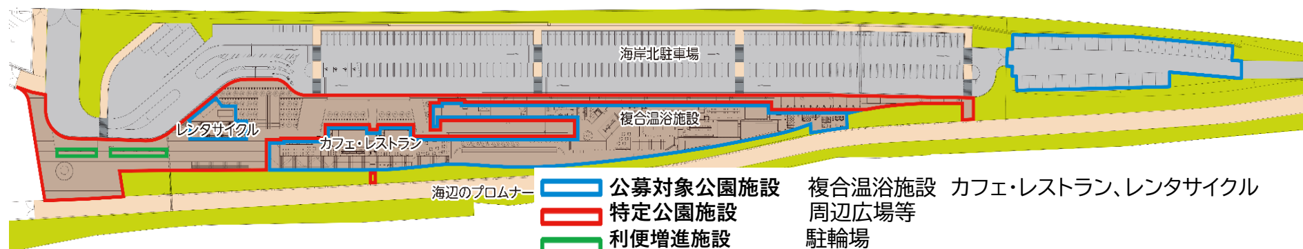
海岸ゾーン「シースケープ・ラウンジ」(2.7ha)平面図
