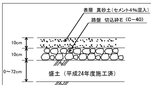
構造図
