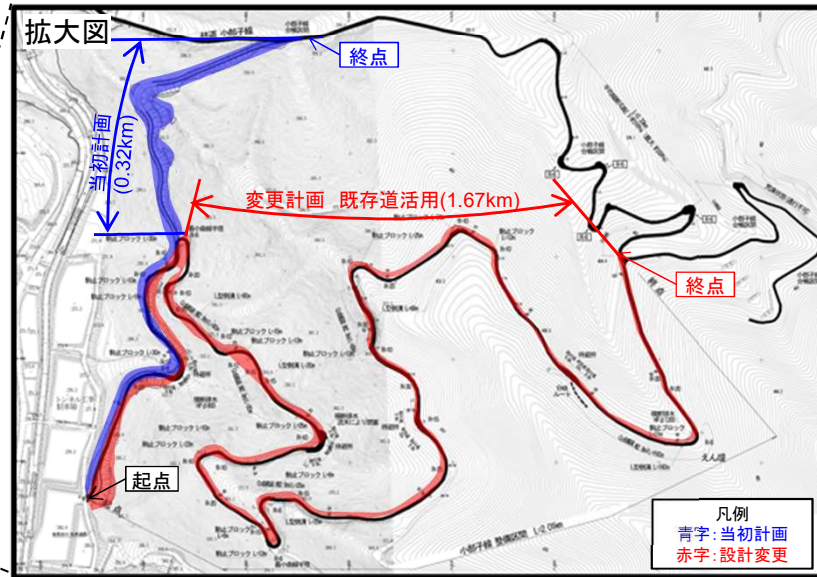
既存道活用区間②
