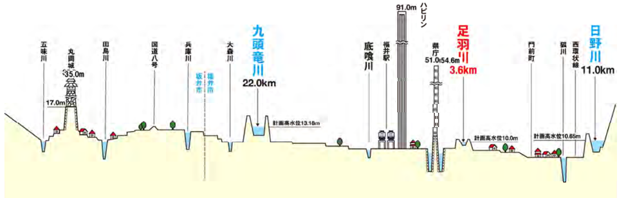
福井市街地断面（洪水時の河川水位は市街地より高い）
