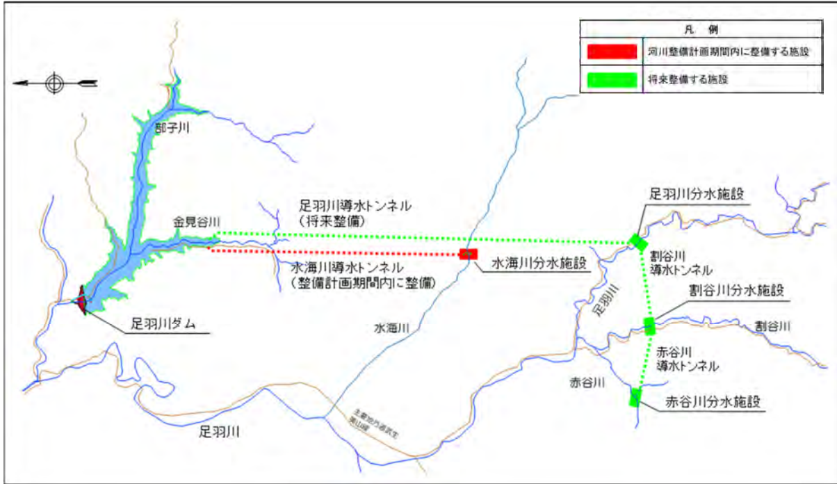
足羽川ダム建設事業 計画平面図（出典：九頭竜川水系河川整備計画）
