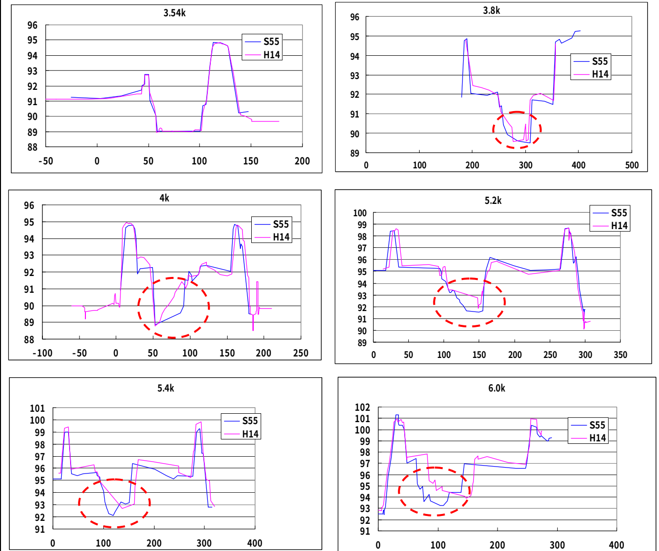
図3-1-2 堆積傾向にある区間の河床高の経年変化(横断面図)
