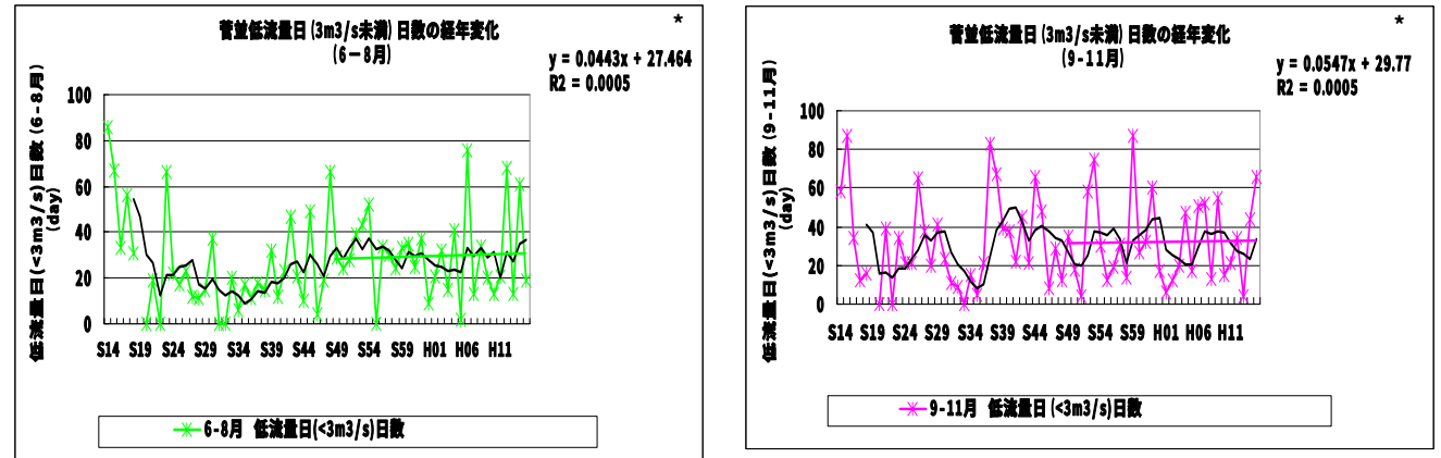
図 3-6 菅並地点における日平均流量 3m³/s 未満の日数の経年変化
