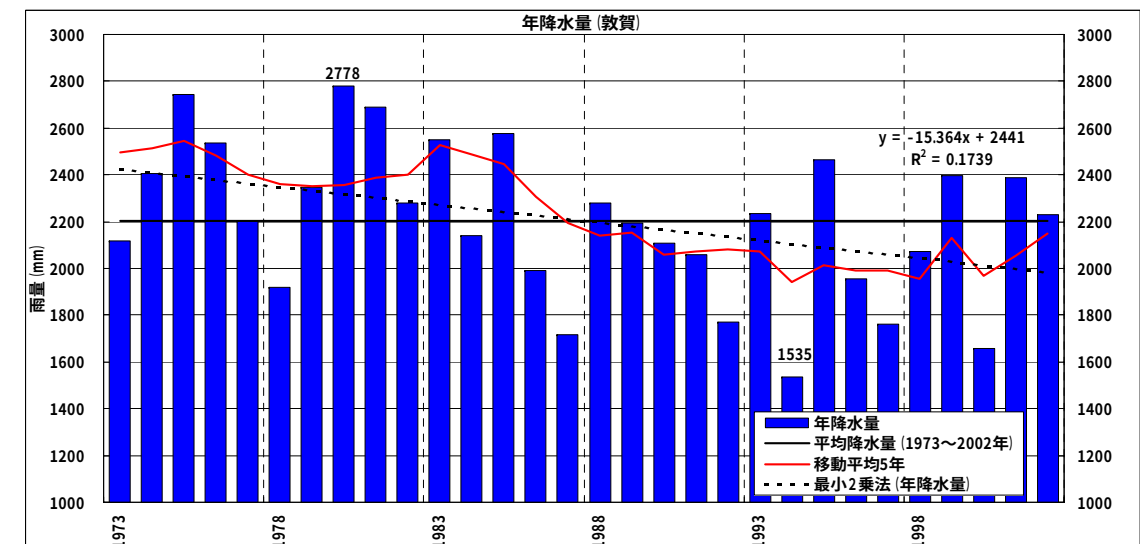
図 3-1 年降水量の経年変化(敦賀)
