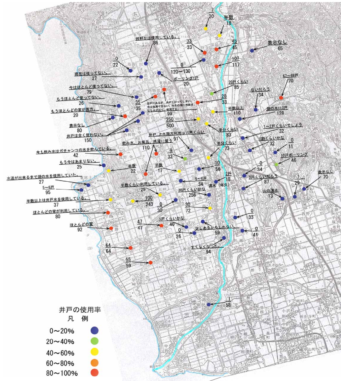
図3-13 高時川沿川の地下水利用状況
