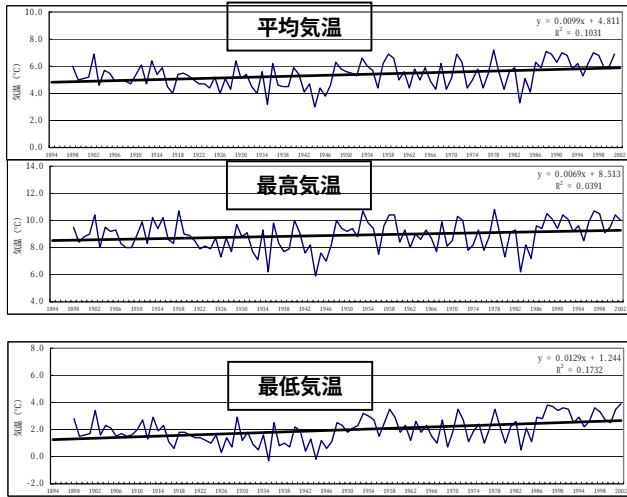
図 3-4-2 冬季気温（敦賀）の経年変化
