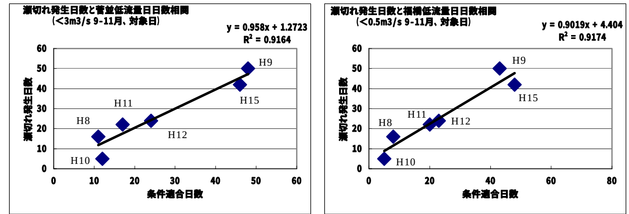
図 3-5 瀬切れ発生日数と低流量日数との相関性
