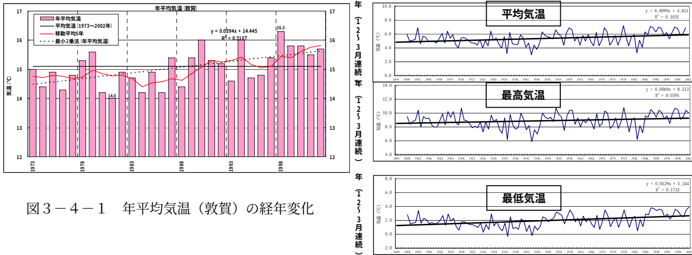
図 3-4-2 冬季気温（敦賀）の経年変化
