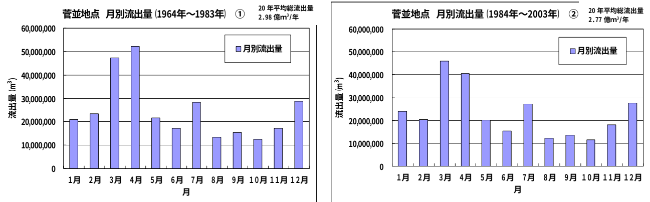
図 3-3 菅並地点の流出量の経年変化
