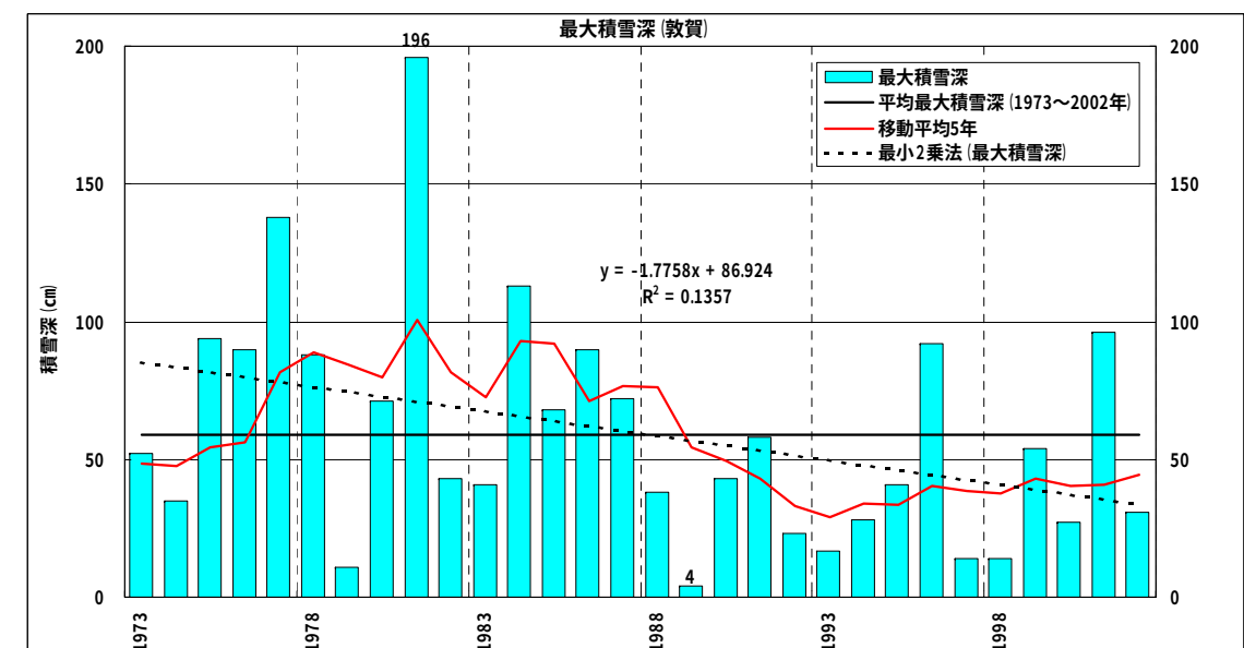
図 3-2 最大積雪深の経年変化 (敦賀)
