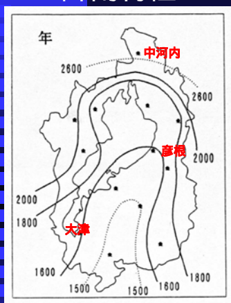
等雨量線図
