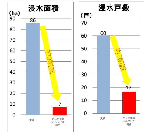
大戸川ダムが整備された場合の 越水による浸水被害の想定
