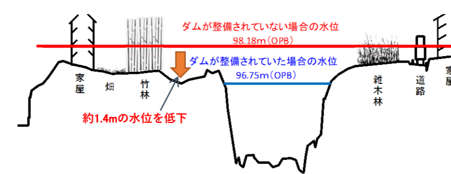
大戸川ダムが整備された場合の 水位低下効果(堂村橋付近)
