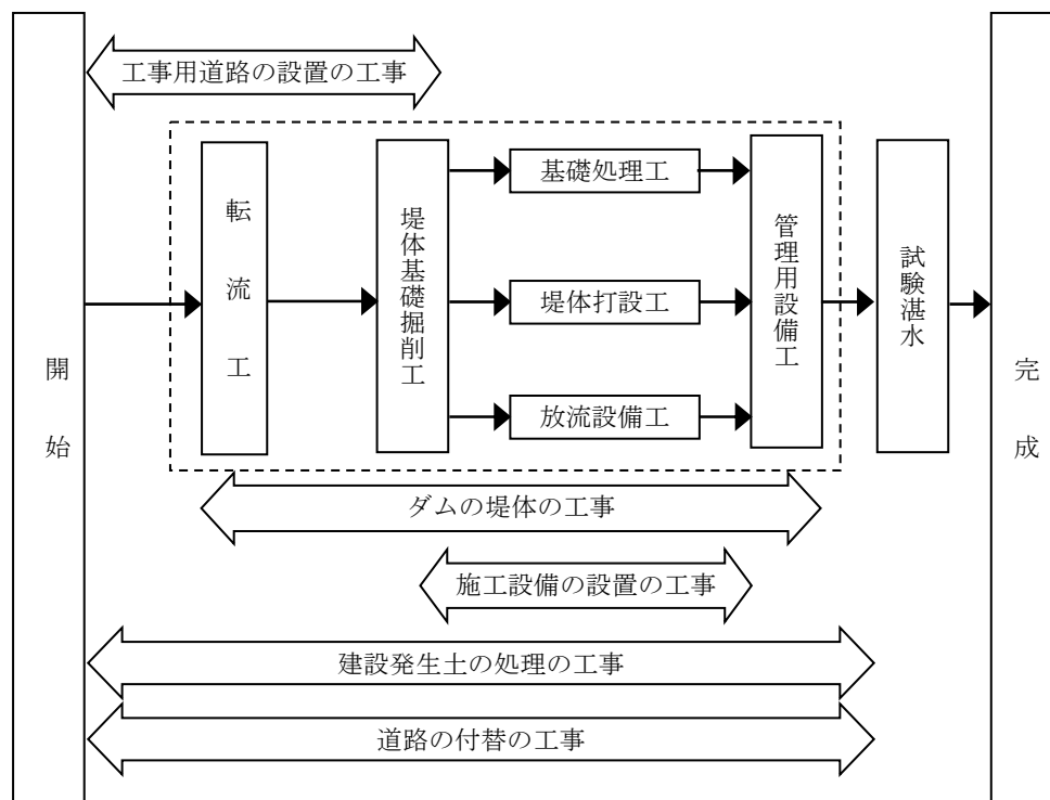
図 1.4-7 工事計画
