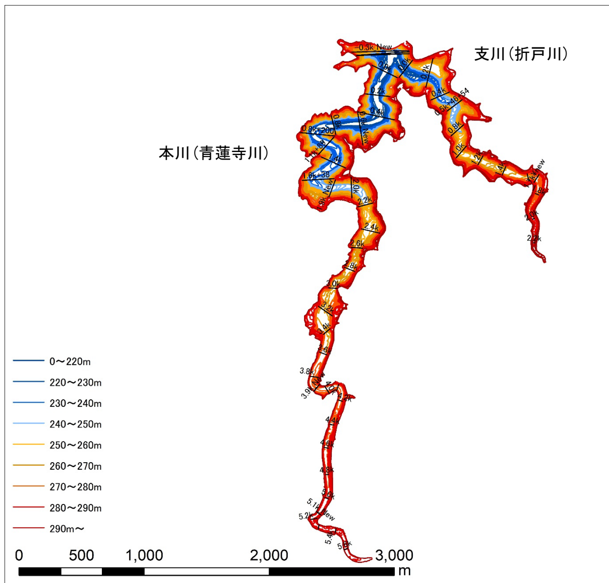
図 5.1.4-37 青蓮寺ダム貯水池の標高区分図
