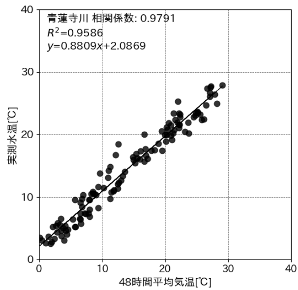
図 5.1.4-38 青蓮寺川（河鹿橋）の実測水温と青蓮寺ダム管理所の48 時間平均気温との関係式
