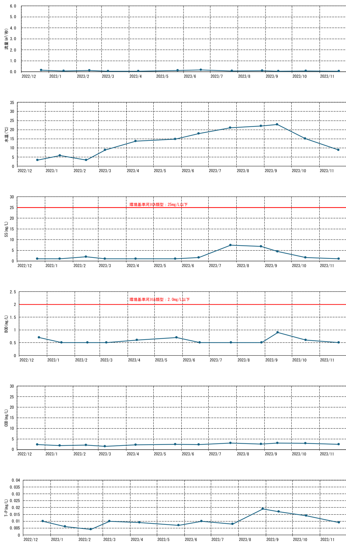
図 5.1.4-7 流入河川（水越川）の定期調査結果（1/3）
