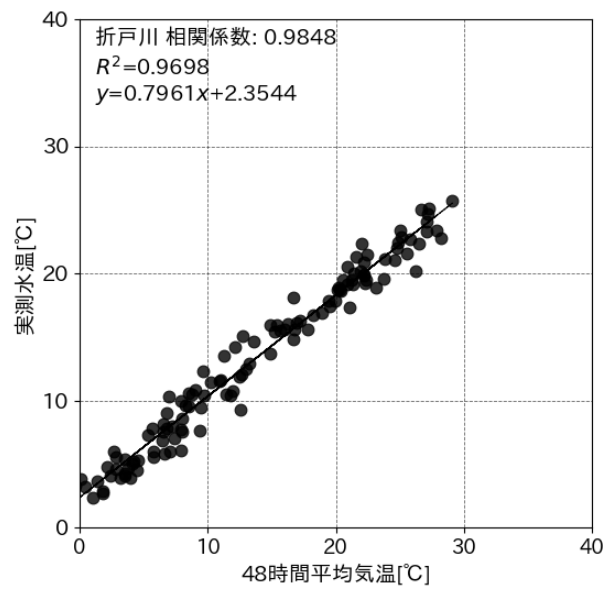
図 5.1.4-39 折戸川（折戸川）の実測水温と青蓮寺ダム管理所の48 時間平均気温との関係式
