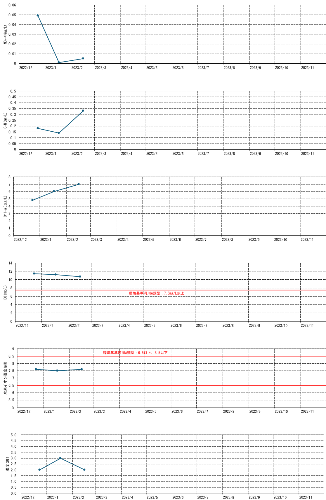
図 5.1.4-12 補足採水地点の定期調査結果 (3/3)
