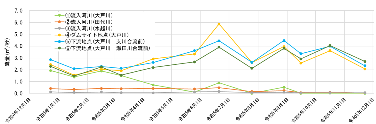
図 5.1.4-4 流量の状況(①流入河川(大戸川)～⑥下流地点(大戸川 瀬田川合流前))
