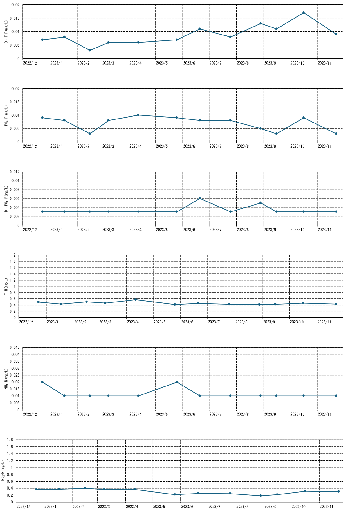
図 5.1.4-8 ダムサイト地点（大戸川）の定期調査結果（2/3）
