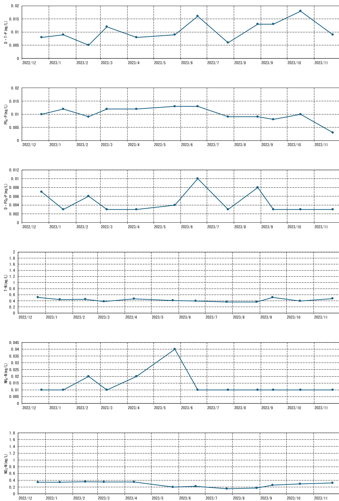
図 5.1.4-5 流入河川（大戸川）の定期調査結果（2/3）
