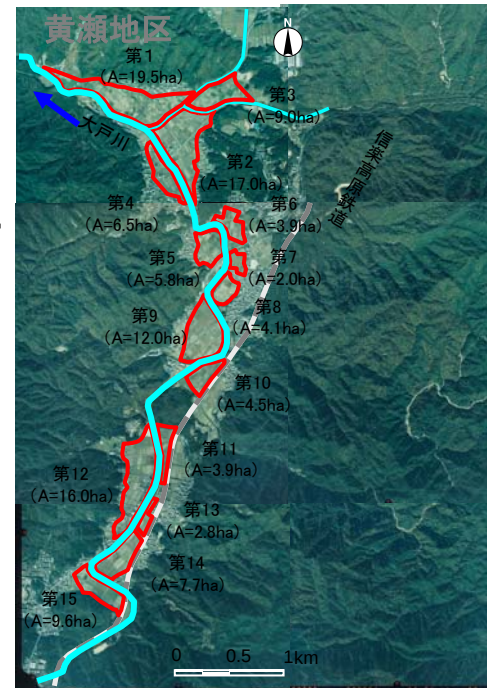
大戸川上流域 確保容量 2,230\text{千m}^3
