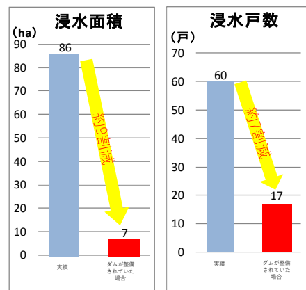
大戸川ダムが整備された場合の 越水による浸水被害の想定
