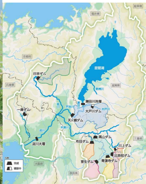
上流の7ダム群の集水面積比較図
