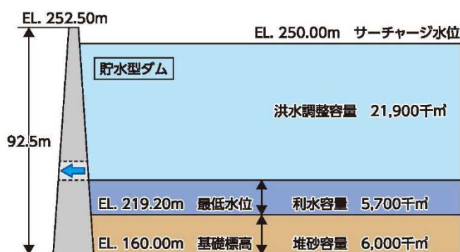
■旧ダム貯水池容量配分図
