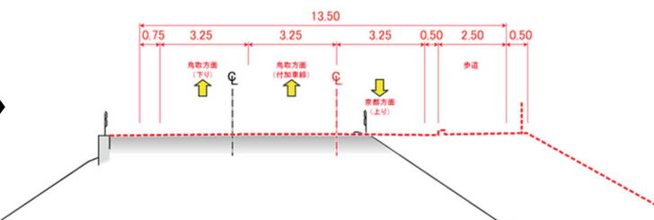
【計画断面図】
