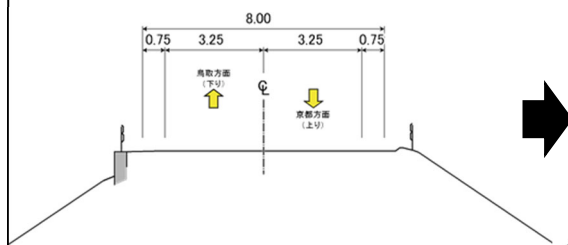
【現況断面図】
