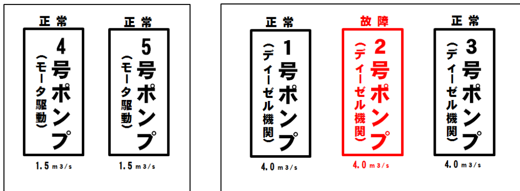
法川排水機場ポンプ配置図
