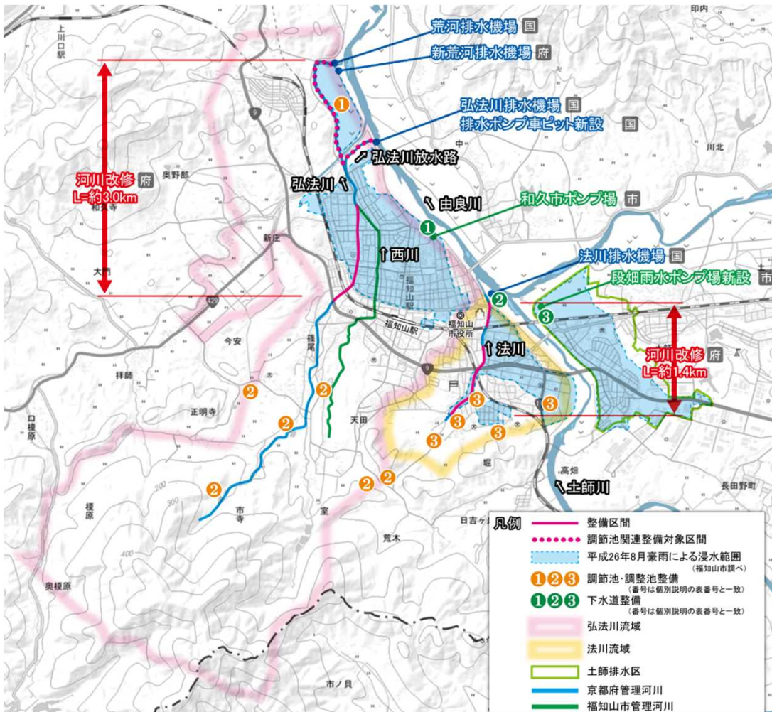
法川排水機場増強(国土交通省)
