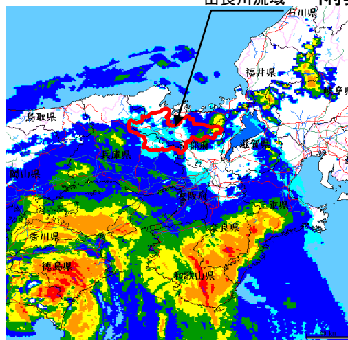
由良川流域 雨雲レーダー
