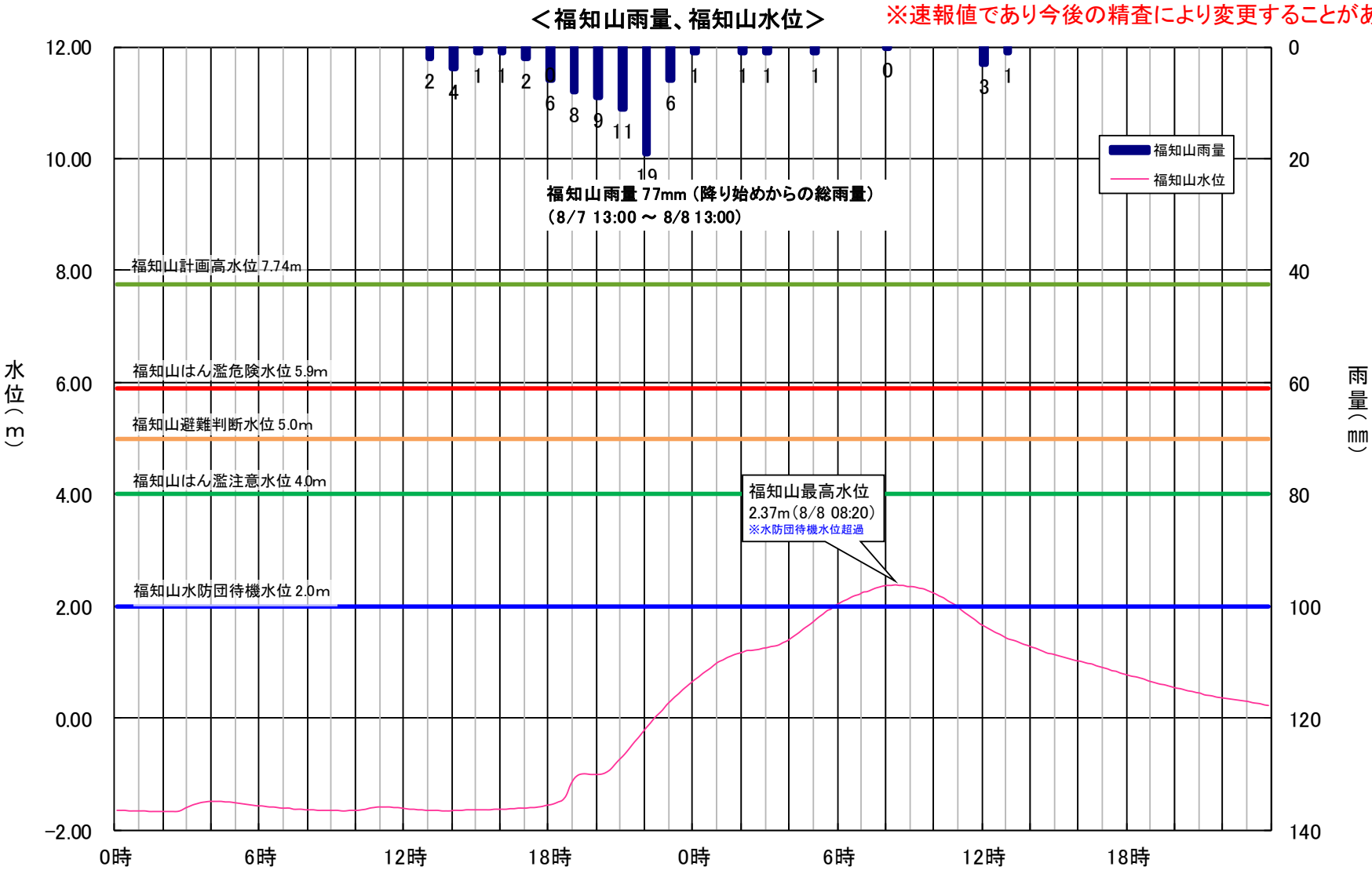
出水概況図（由良川水系 H29. 8. 7～H29. 8. 8）
