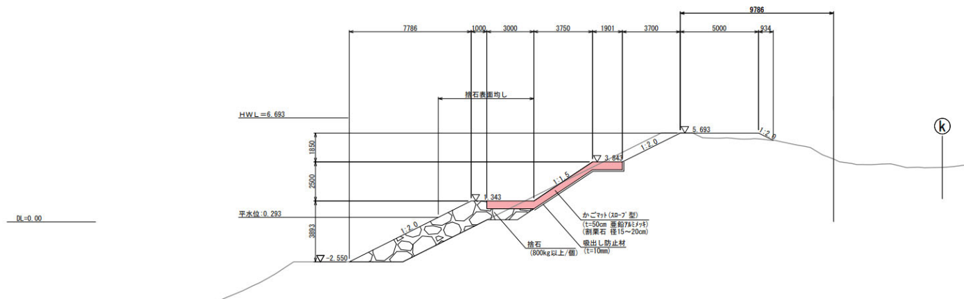
標準断面図
