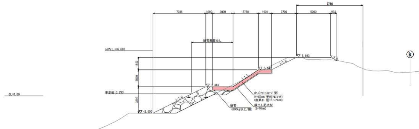
標準断面図
