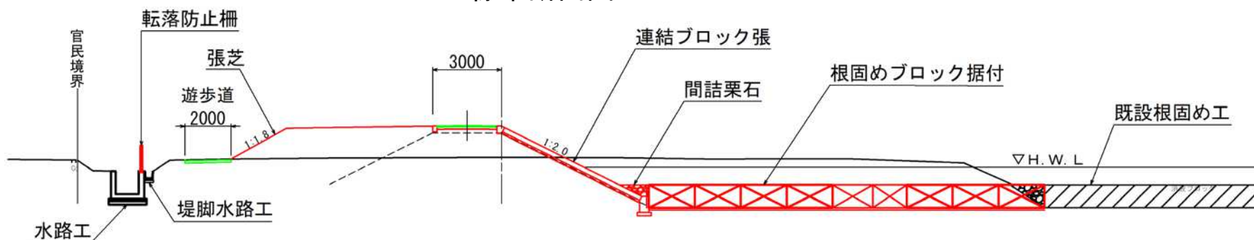
標準断面図
