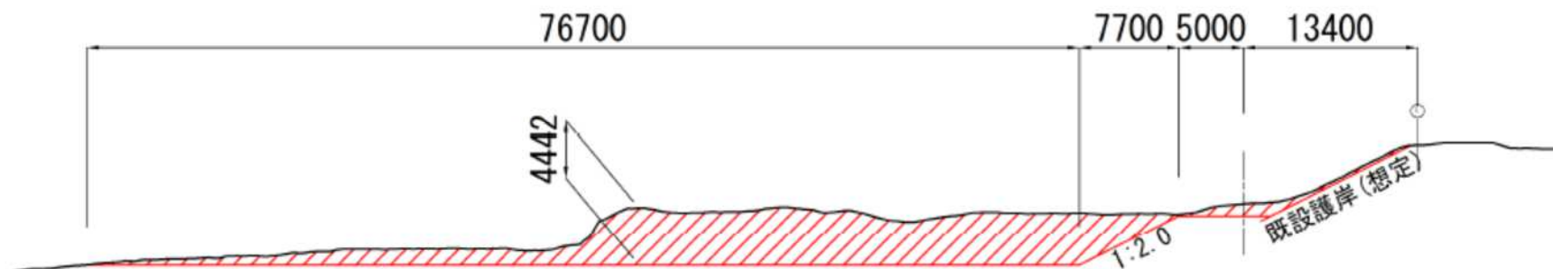
標準断面図
