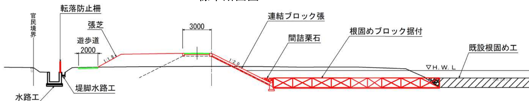
標準断面図
