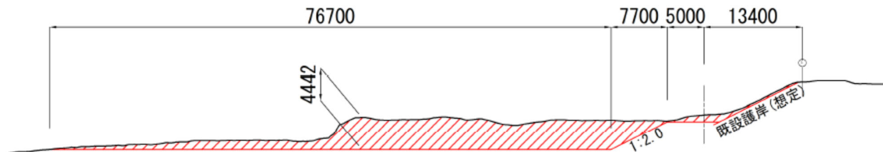
標準断面図
