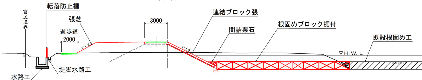
標準断面図
