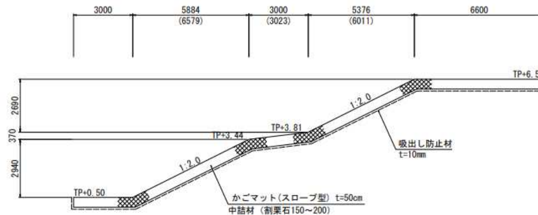
標準断面図
