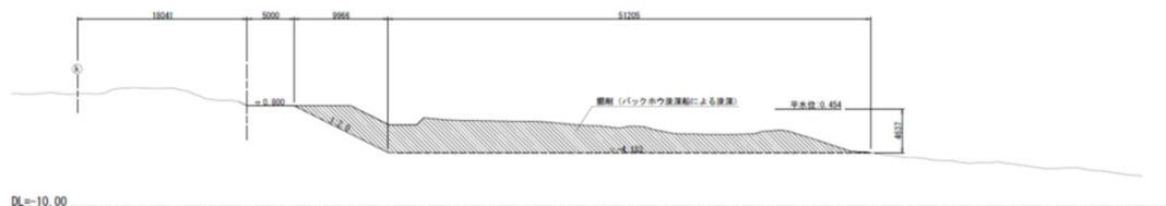
標準断面図
