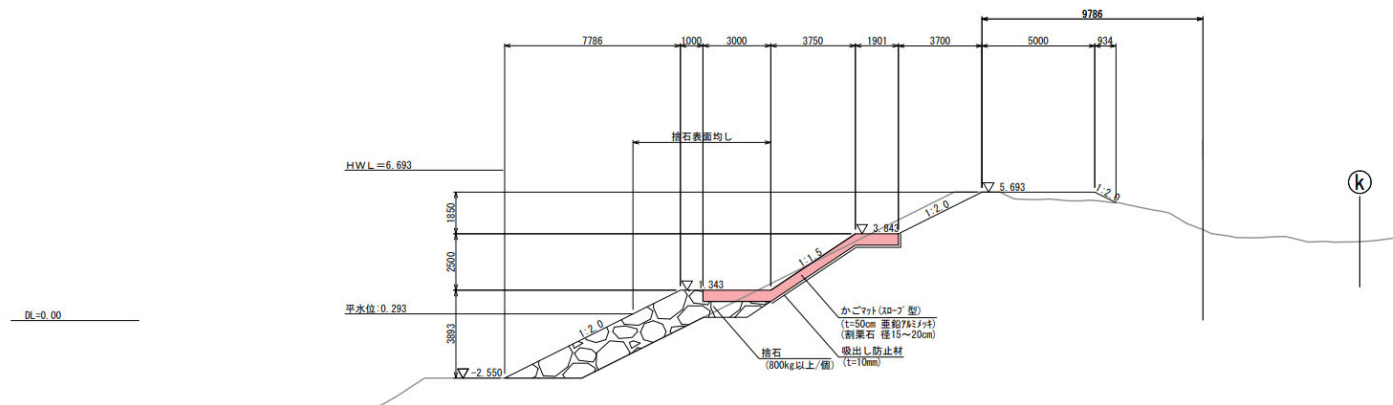
標準断面図
