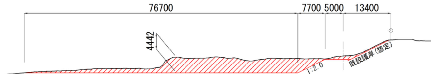
標準断面図
