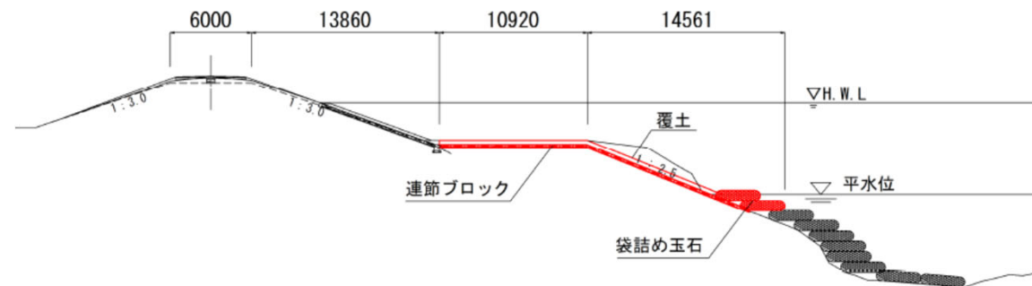
標準断面図
