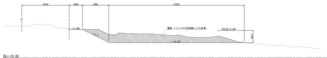
標準断面図
