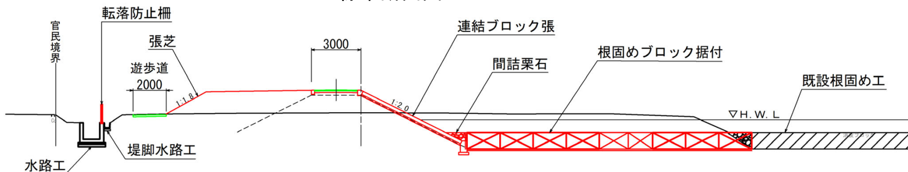
標準断面図
