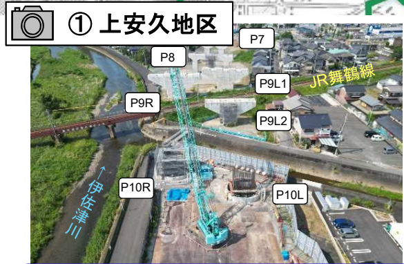
上安久高架橋(仮称)のP10R・L橋脚のケーソン基礎が概ね完了し、橋脚鉄筋の立ち上げ、足場を設置しています。
