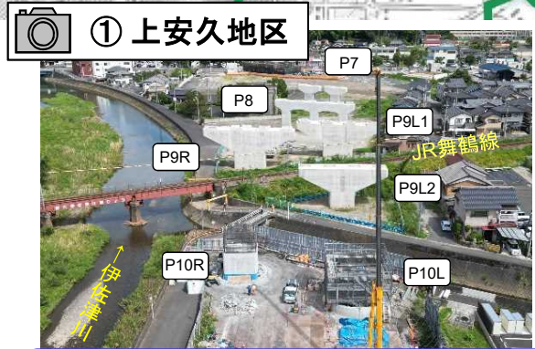
上安久高架橋(仮称)のP10R・L橋脚のケーソン基礎は概ね完了。P10Rは橋脚の梁部を除きコンクリート打設完了、P10Lは鉄筋組立中です。
