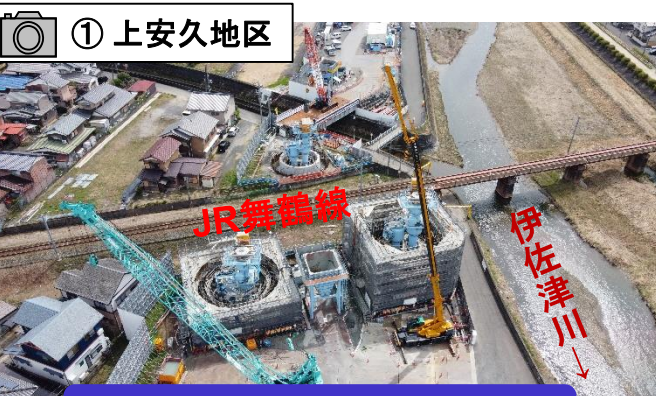
高架橋下部工事のケーソン基礎工を実施
