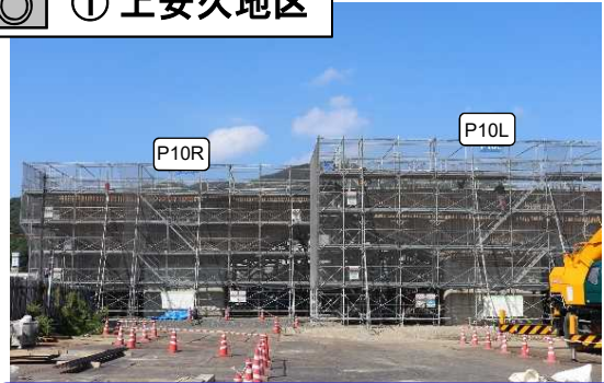
上安久高架橋(仮称)のP10R橋脚はコンクリートの打ち込みが完了。P10L橋脚は鉄筋の組立が完了しました。
