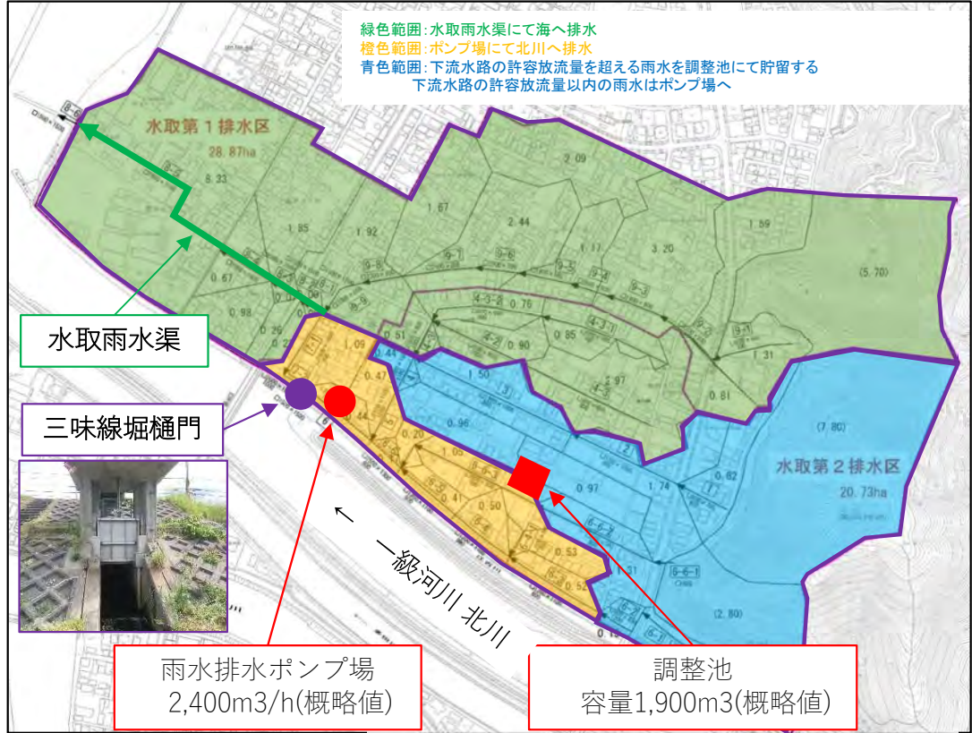
平面図 (水取排水区 A=49.6ha)
