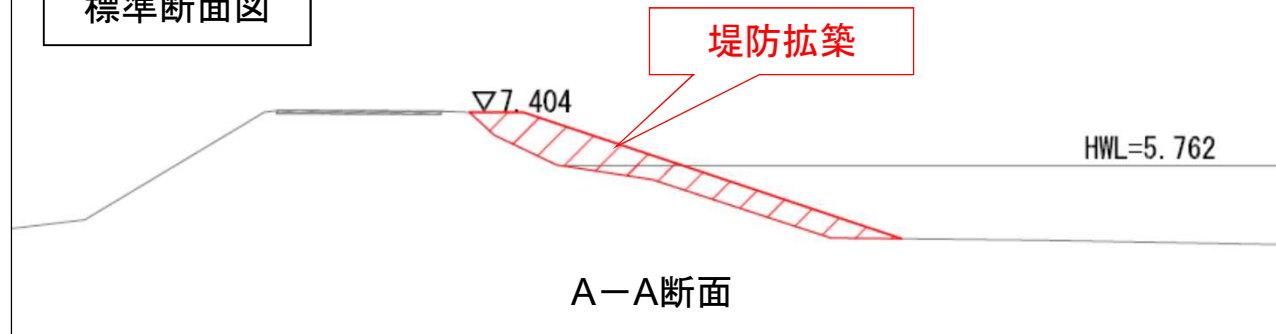
標準断面図
