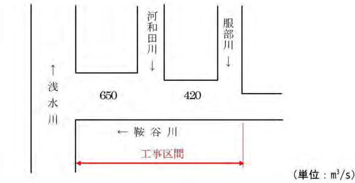
図 5.22 計画流量配分図
