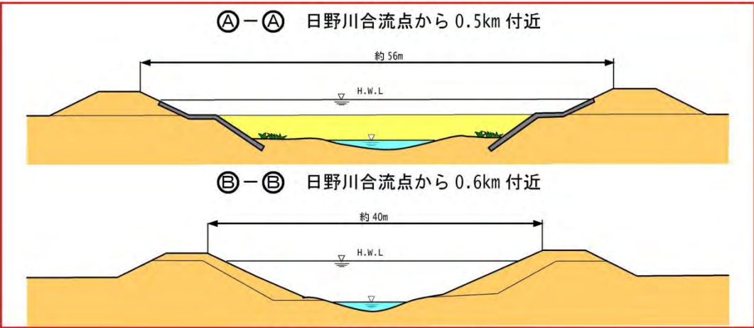
図 5.30 横断面図（イメージ）
