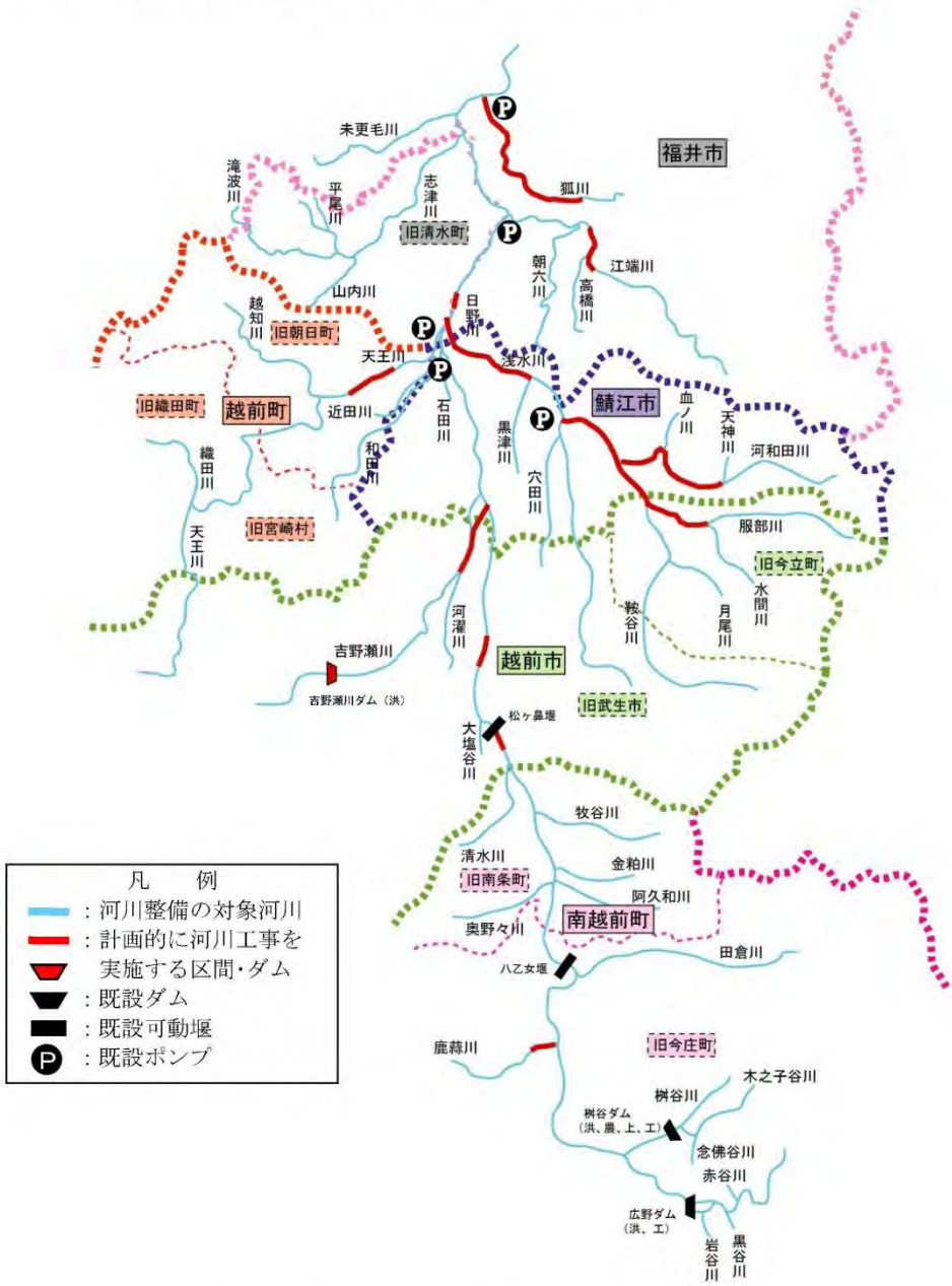
図 5.1 計画的に河川工事を実施する区間
