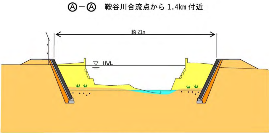
図 5.20 横断面図（イメージ）
