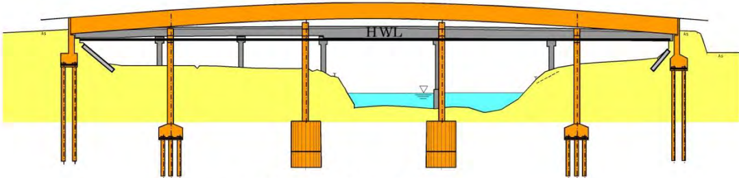
図 5.4 横断面図（イメージ）
