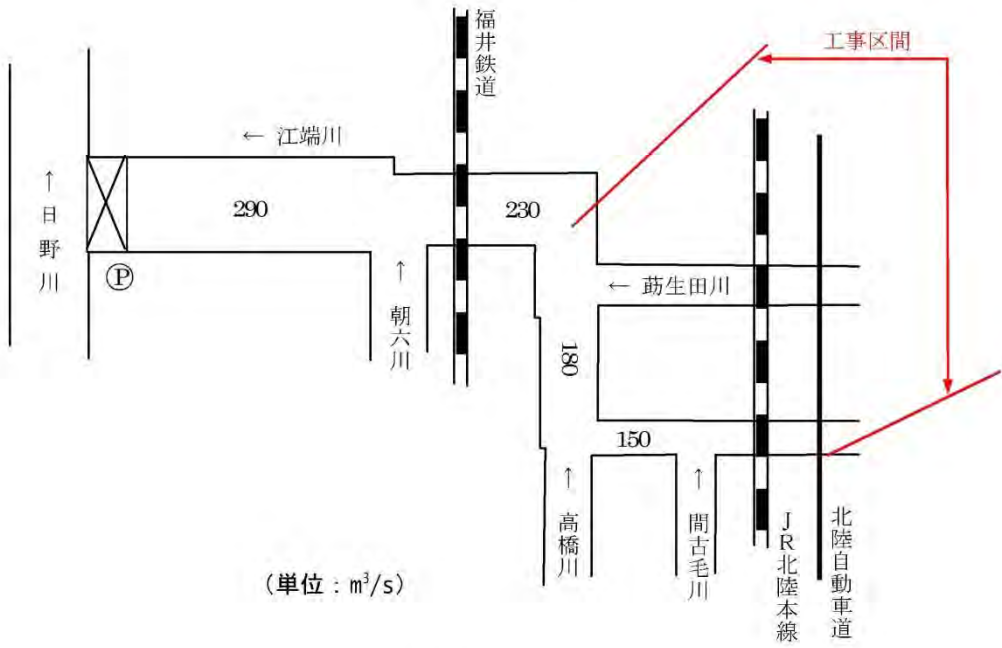
図 5.16 計画流量配分図
