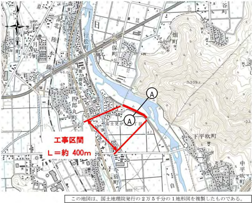
図 5.7 平面図
