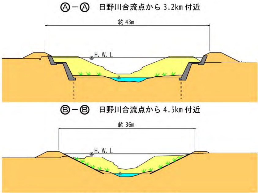
図 5.11 横断面図（イメージ）
