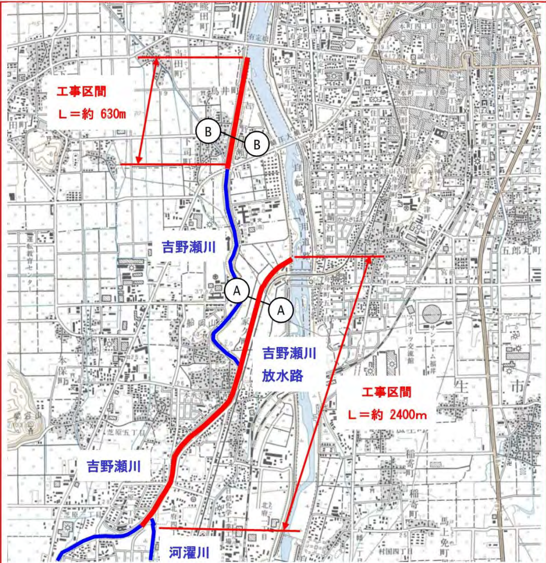
図 5.29 平面図
