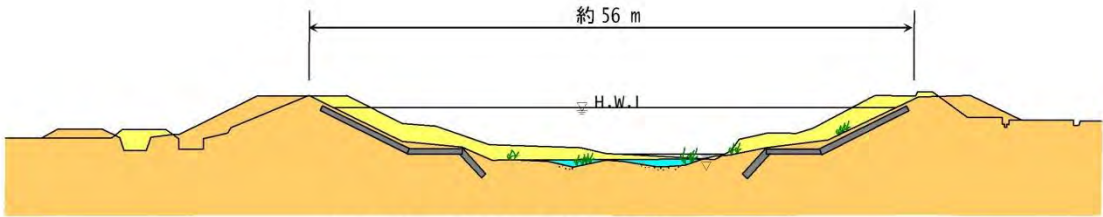
図 5.35 横断面図（イメージ）
