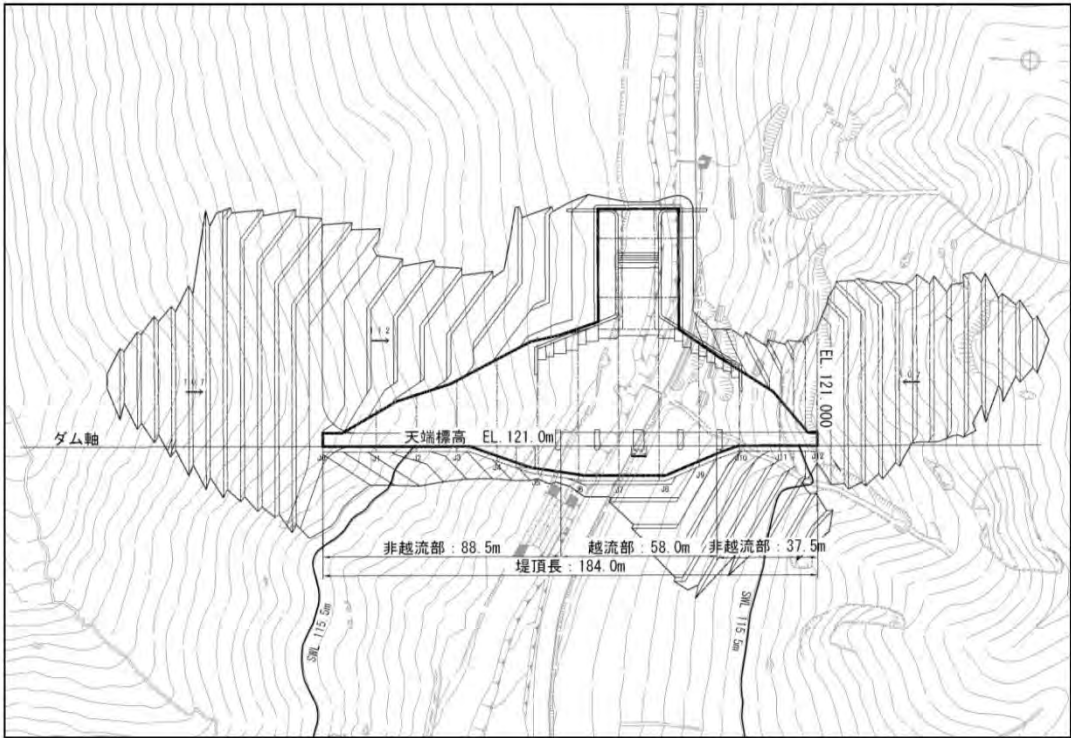
図 5.39 平面図
