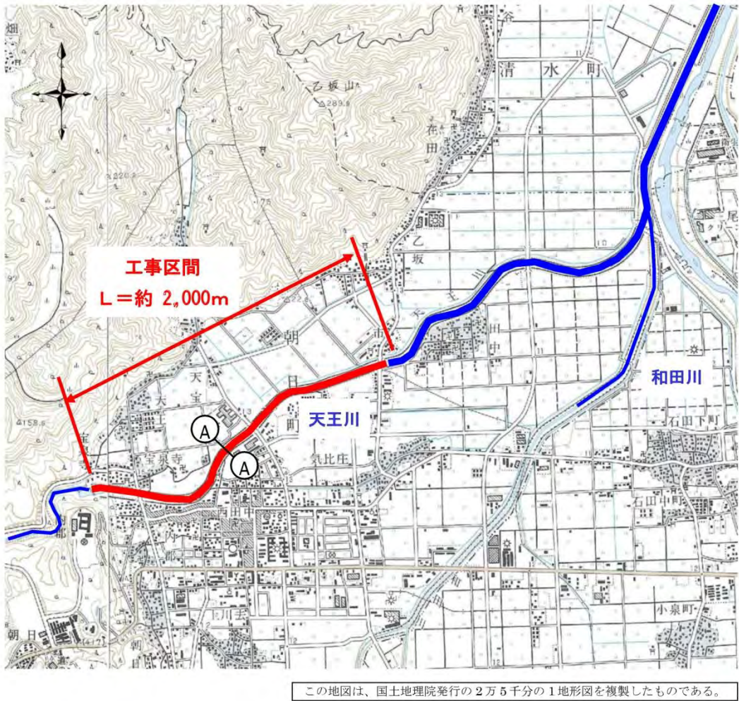
図 5.22 平面図
