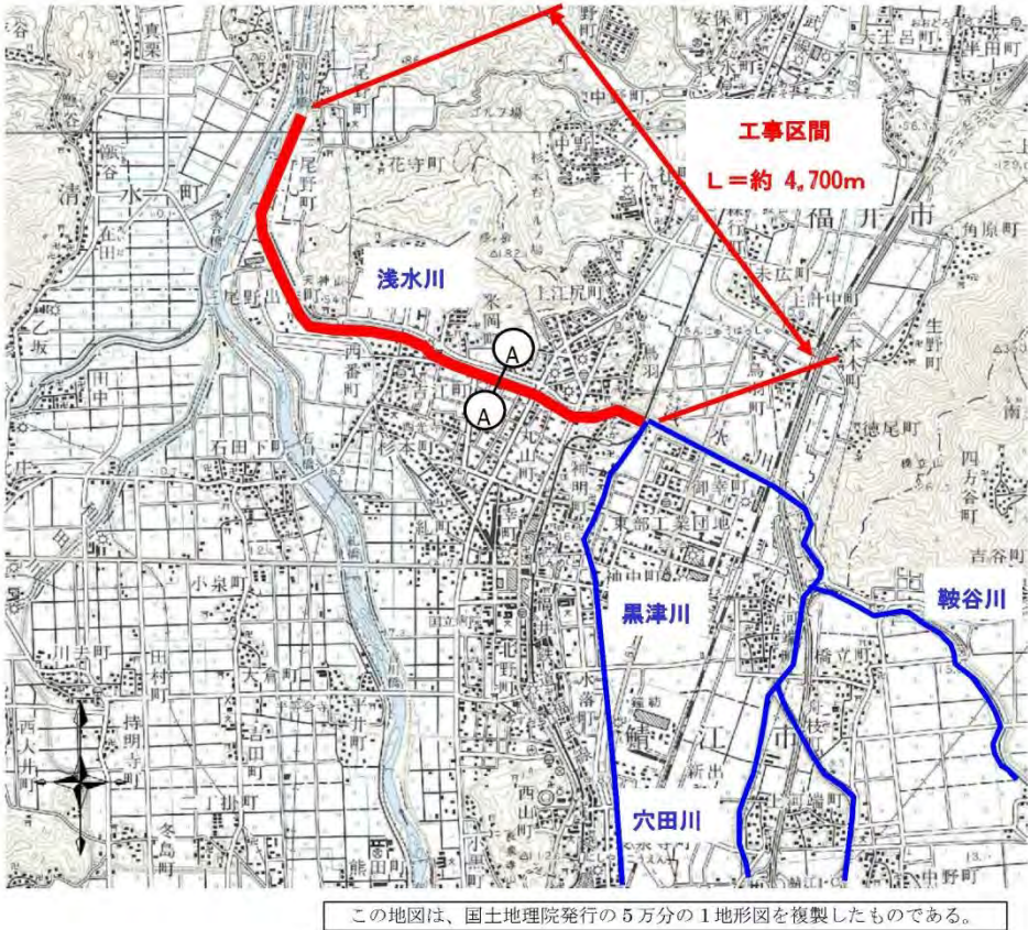
図 5.20 平面図
