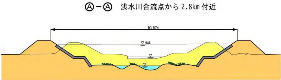
図 5.14 横断面図（イメージ）
