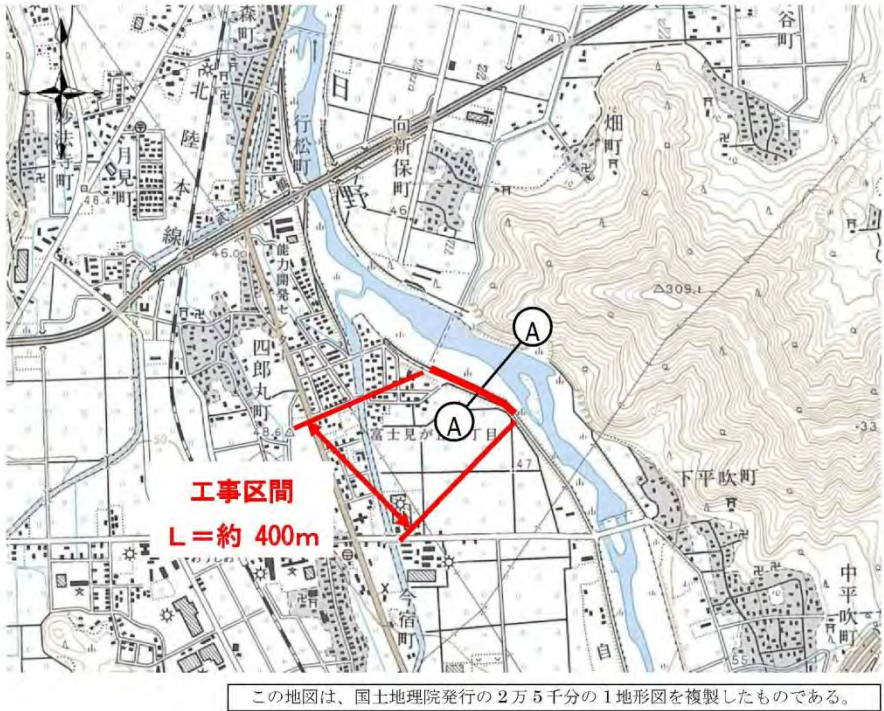
図 5.7 平面図
