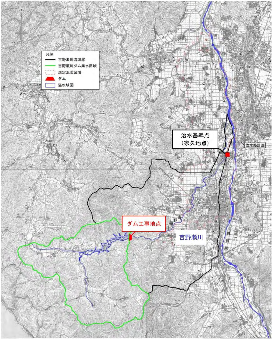
図 5.38 ダム位置図
