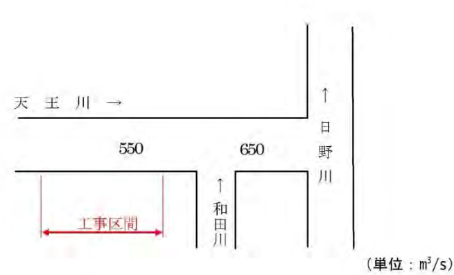
図 5.33 計画流量配分図
