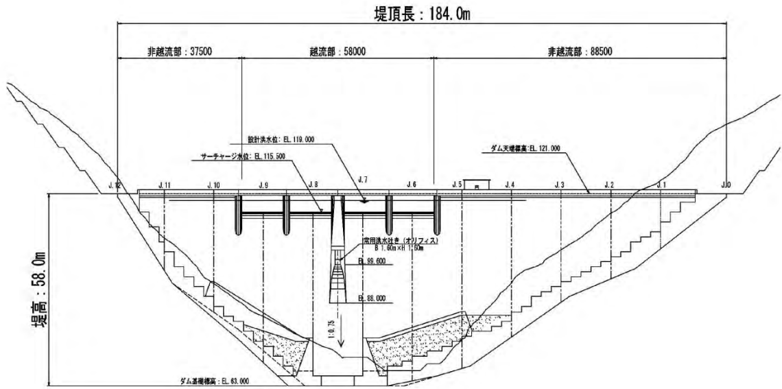
図 5.40 下流面図
