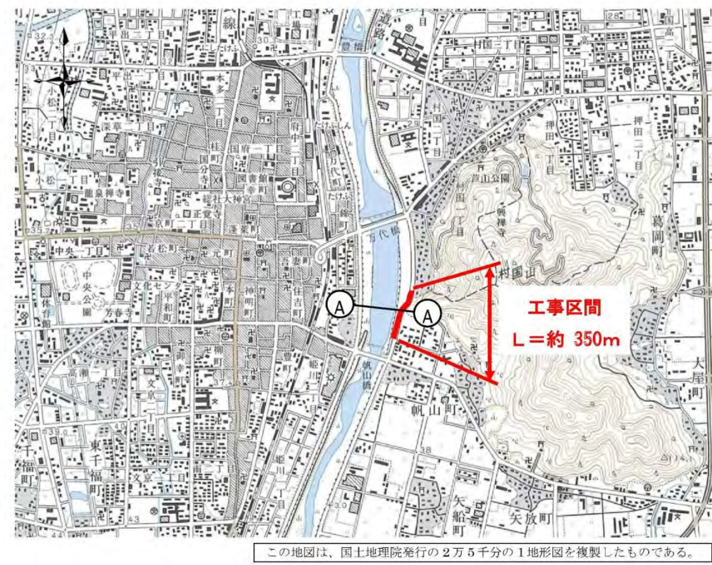
図 5.5 平面図
