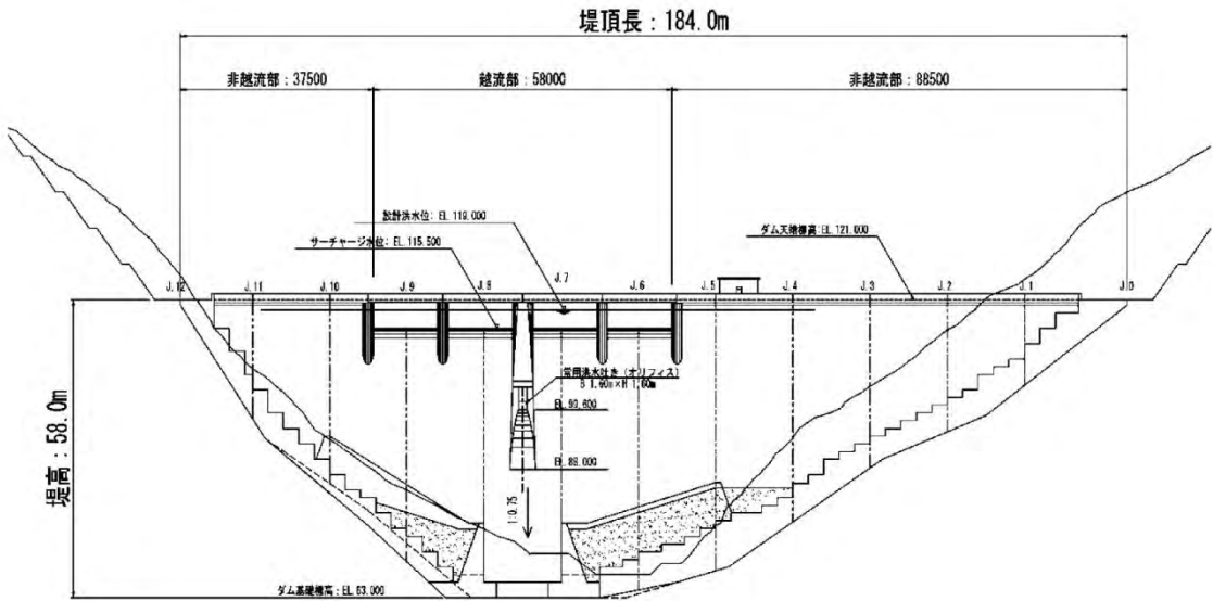
図 5.28 下流面図
