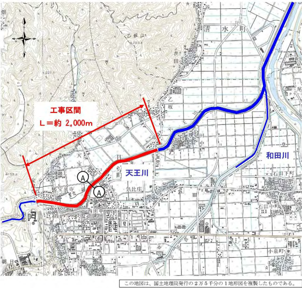
図 5.34 平面図
