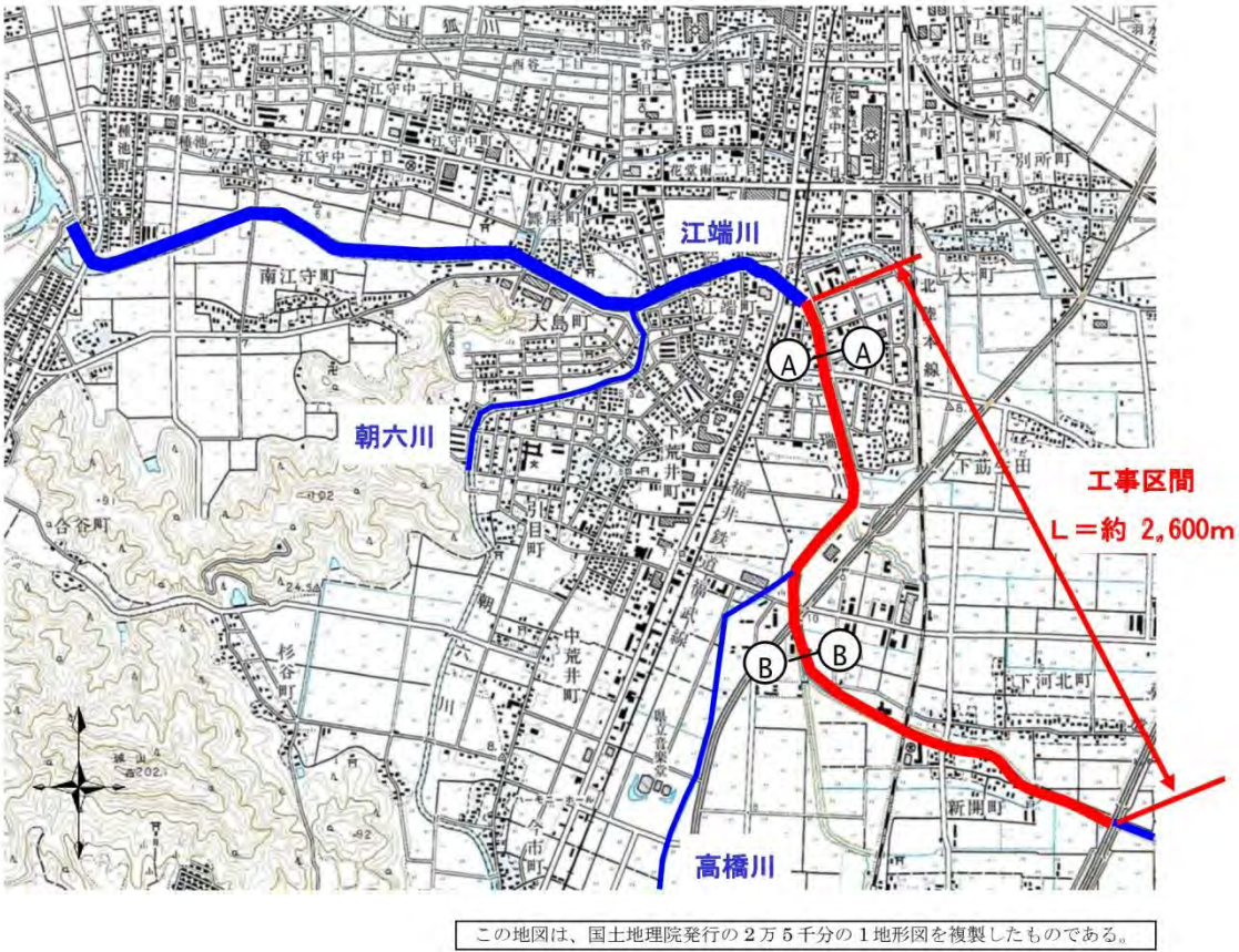
図 5.10 平面図
