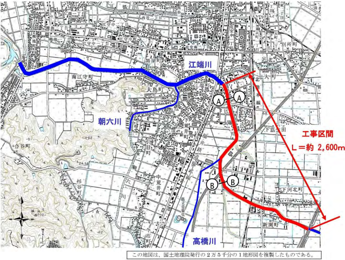
図 5.17 平面図
