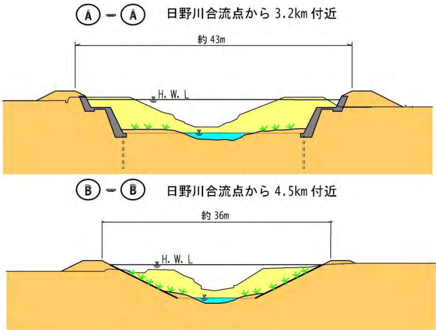
図 5.18 横断面図（イメージ）
