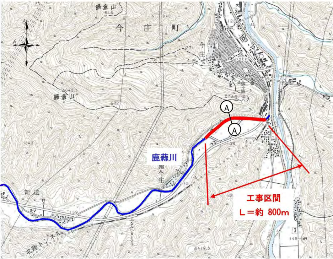
図 5.44 平面図
