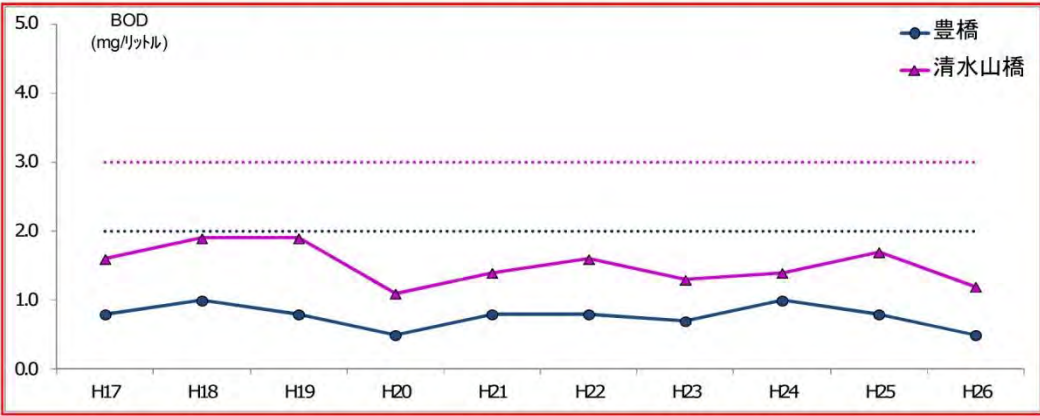
図 3.1 日野川の水質（BOD75%値）の推移
