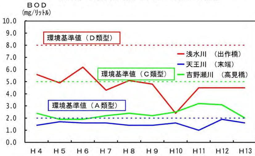
図 3.2 支川の水質（BOD75%値）の推移
