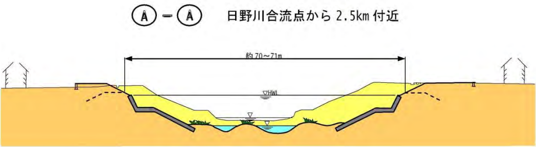
図 5.21 横断面図（イメージ）
