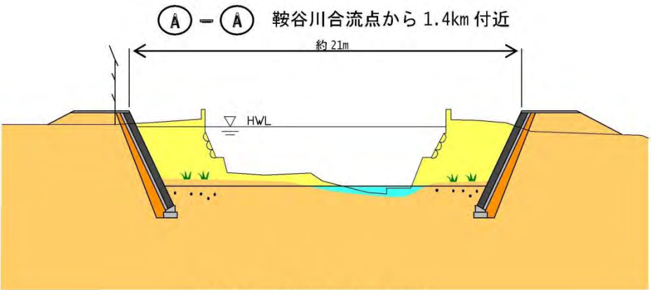
図 5.32 横断面図（イメージ）
