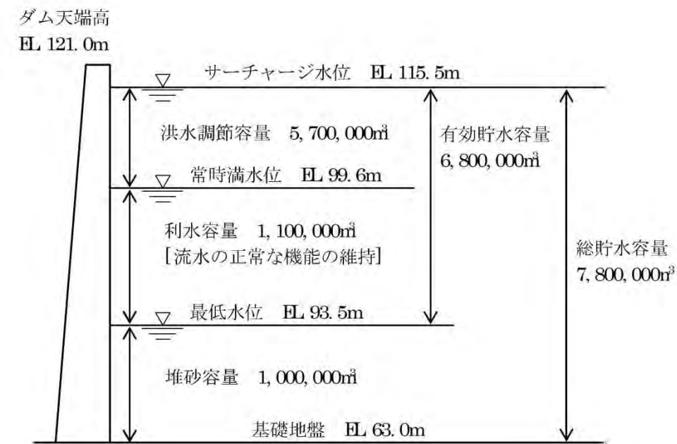
図 5.37 ダム容量配分図
