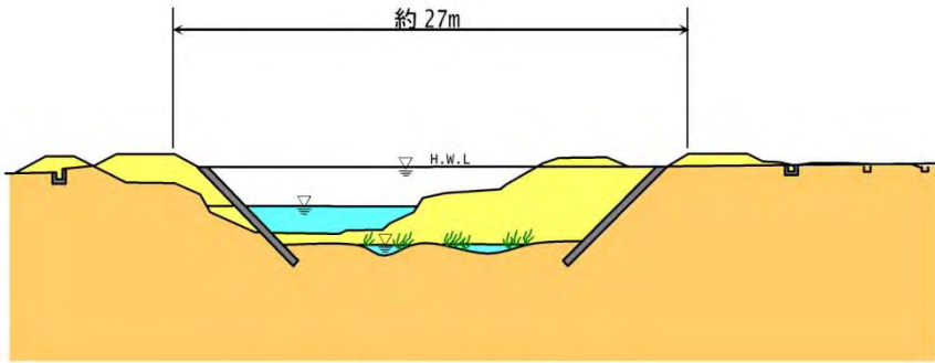
図 5.17 横断面図（イメージ）
