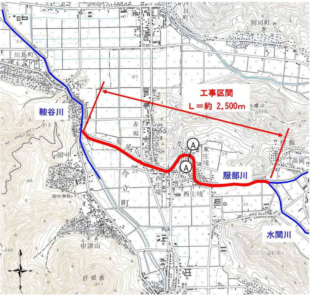
図 5.31 平面図
