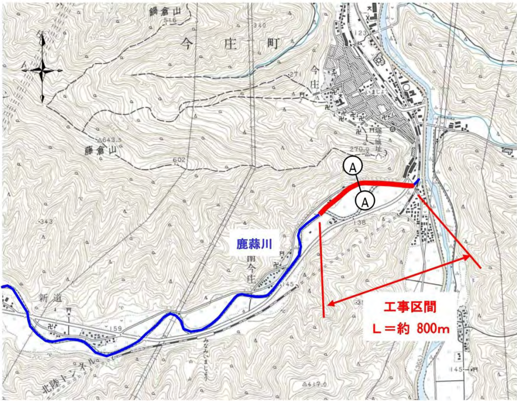
図 5.32 平面図
