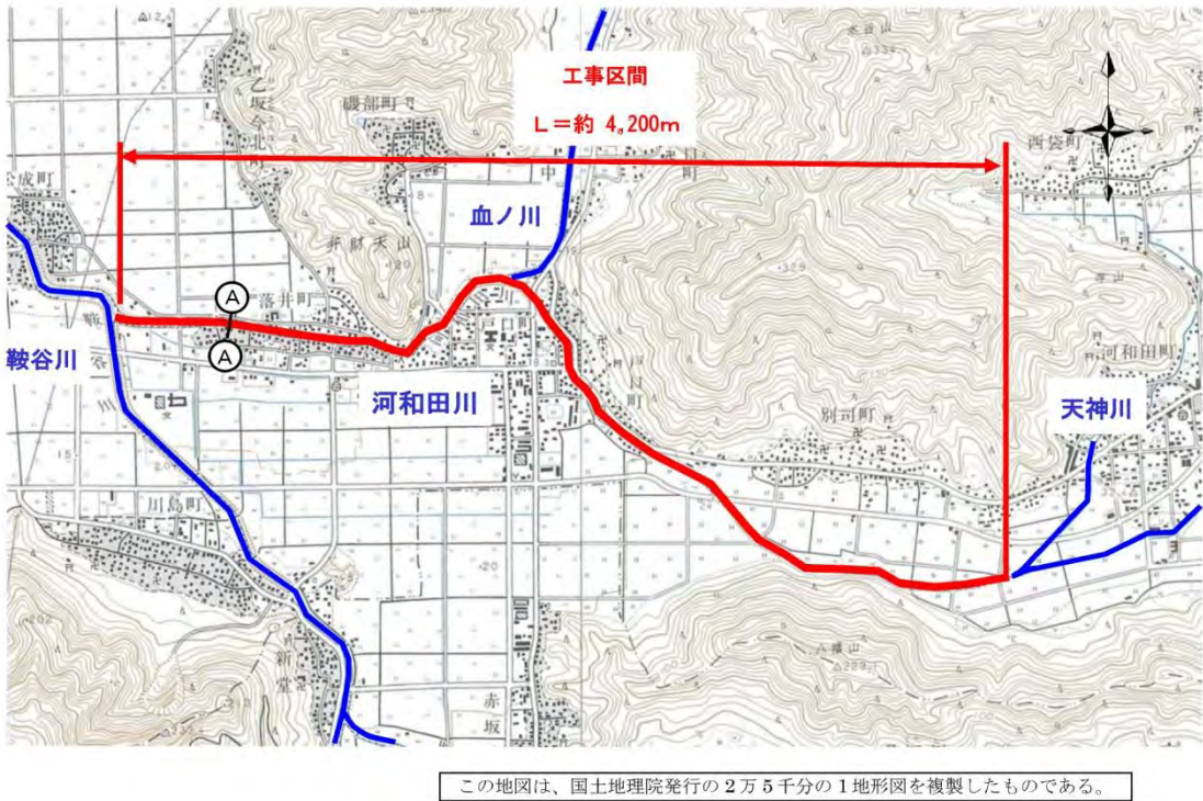
図 5.16 平面図
