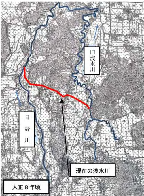
図 2.1 浅水川の新川開削区間
