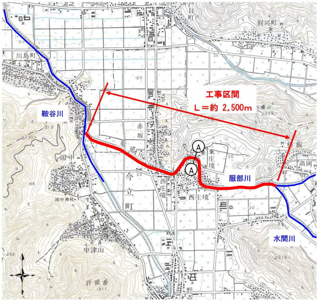
図 5.19 平面図
