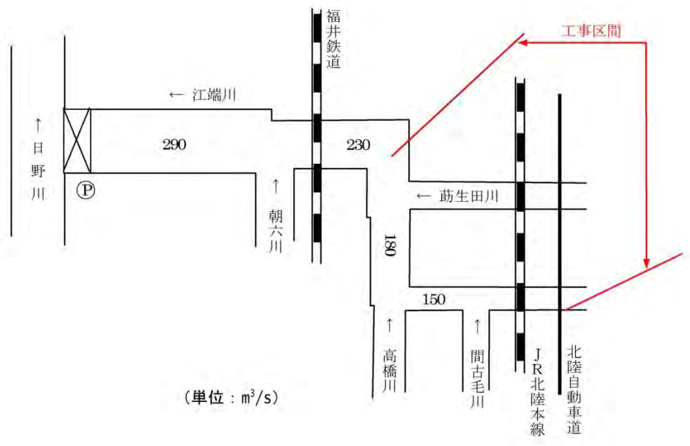
図 5.9 計画流量配分図
