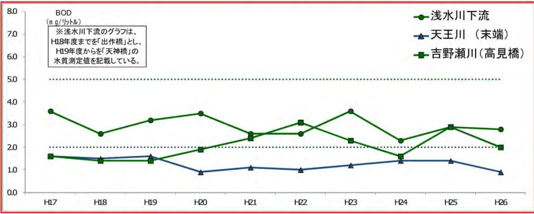
図 3.2 支川の水質（BOD75%値）の推移
