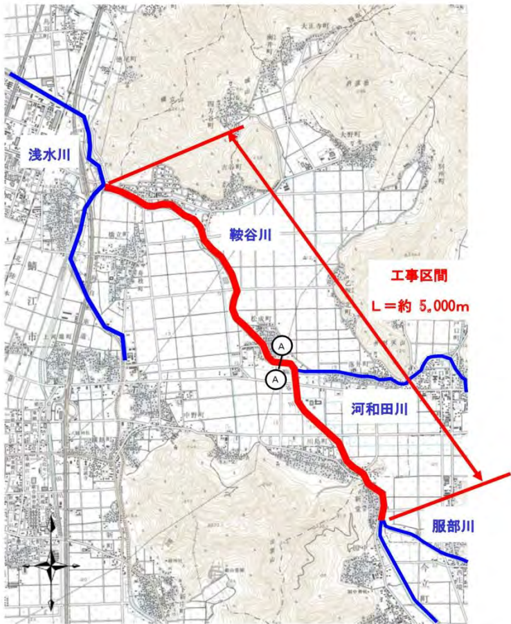
図 5.13 平面図
