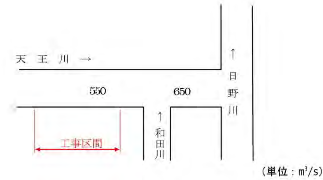
図 5.21 計画流量配分図
