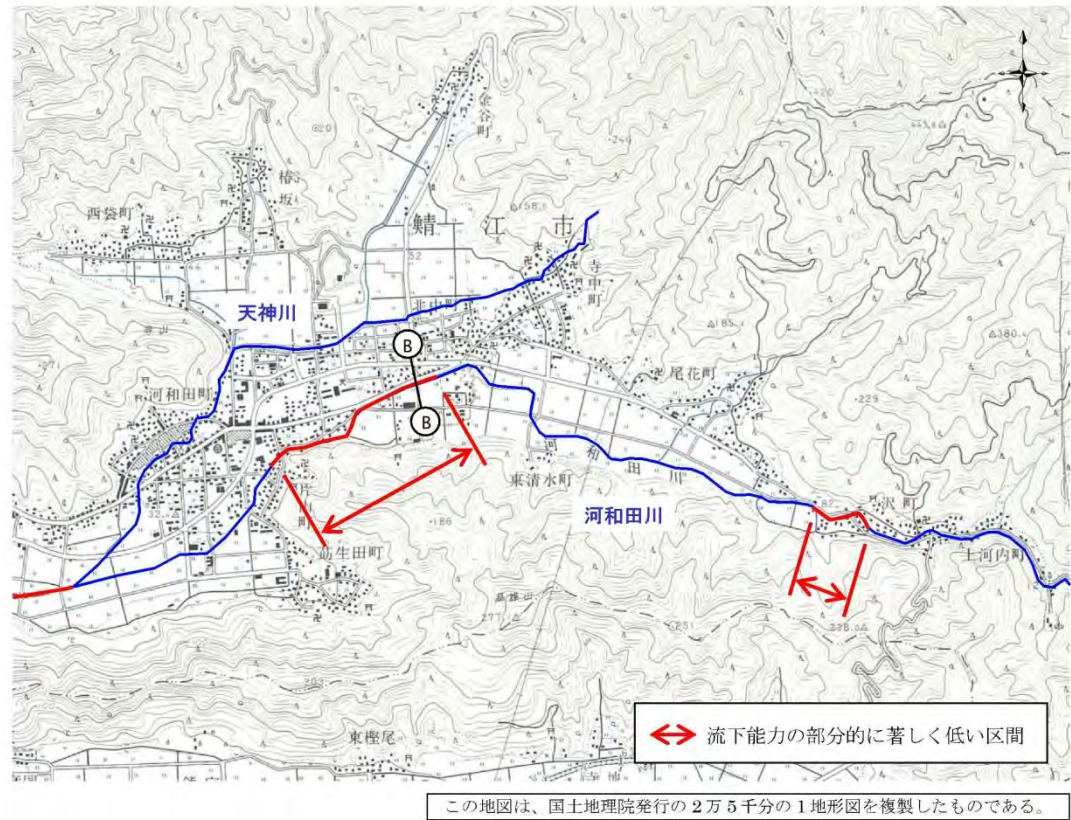
図 5.28 平面図
