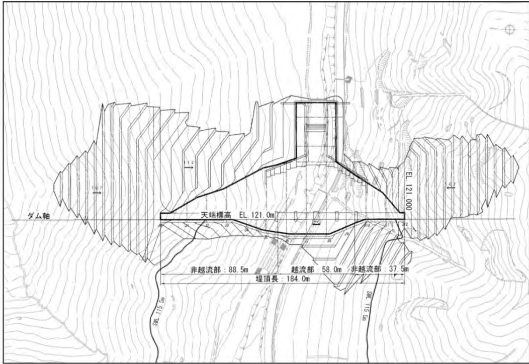
図 5.27 平面図
