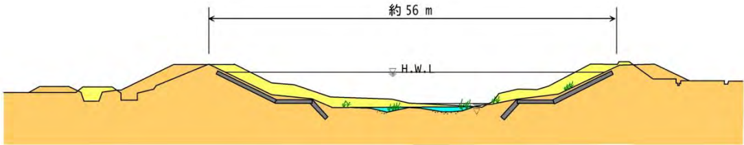
図 5.23 横断面図（イメージ）
