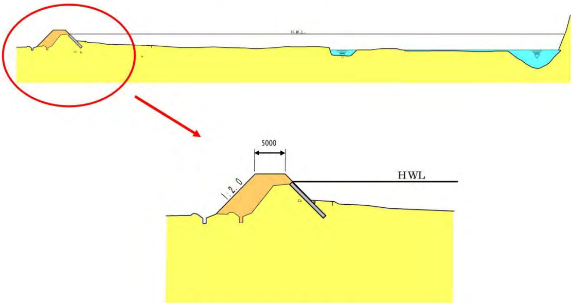
図 5.8 横断面図（イメージ）
