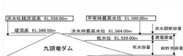
九頭竜ダムの容量配分図
