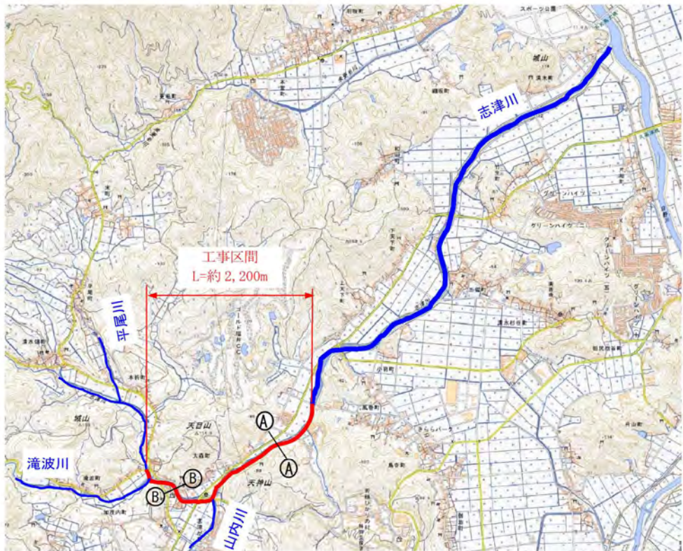
図 5.10 平面図
