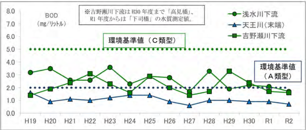
図 3.2 支川の水質（BOD75%値）の推移
