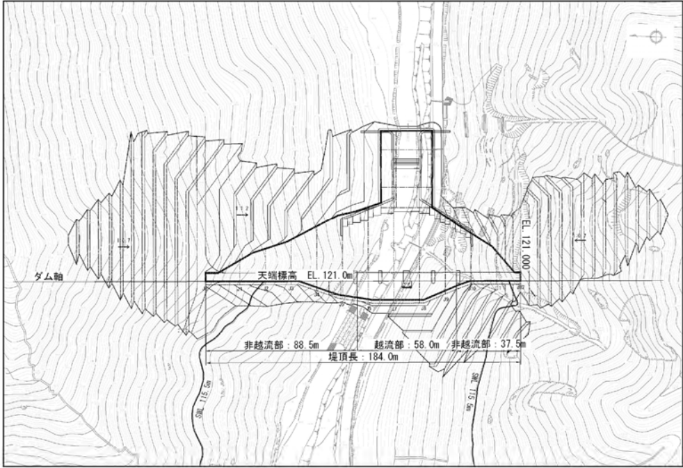
図 5.27 平面図
