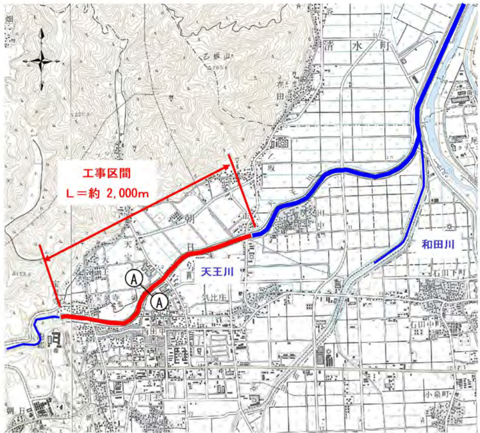
図 5.22 平面図
