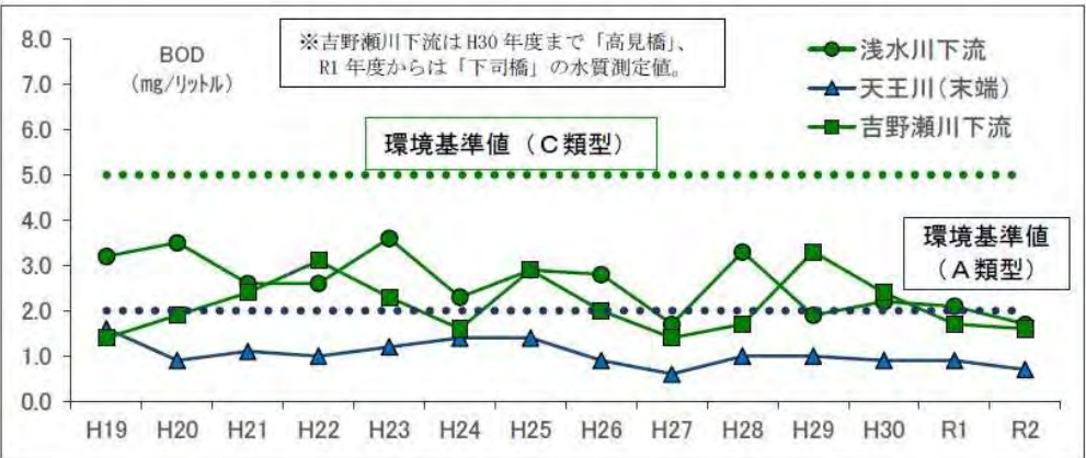
図 3.2 支川の水質（BOD75%値）の推移
