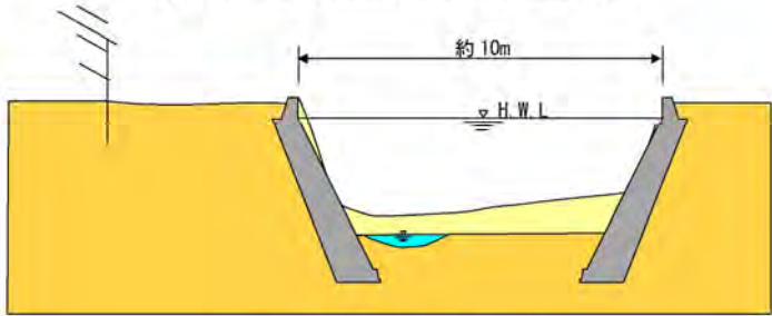
図 5.11 横断面図（イメージ）
