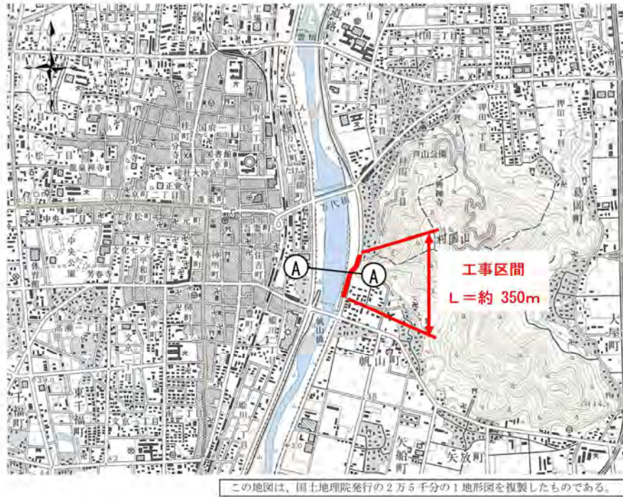
図 5.5 平面図
