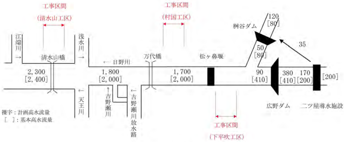
図 5.2 計画流量配分図
