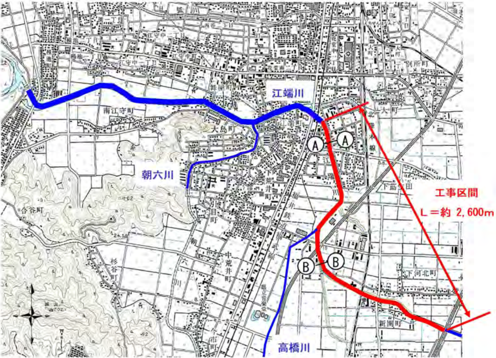
図 5.13 平面図
