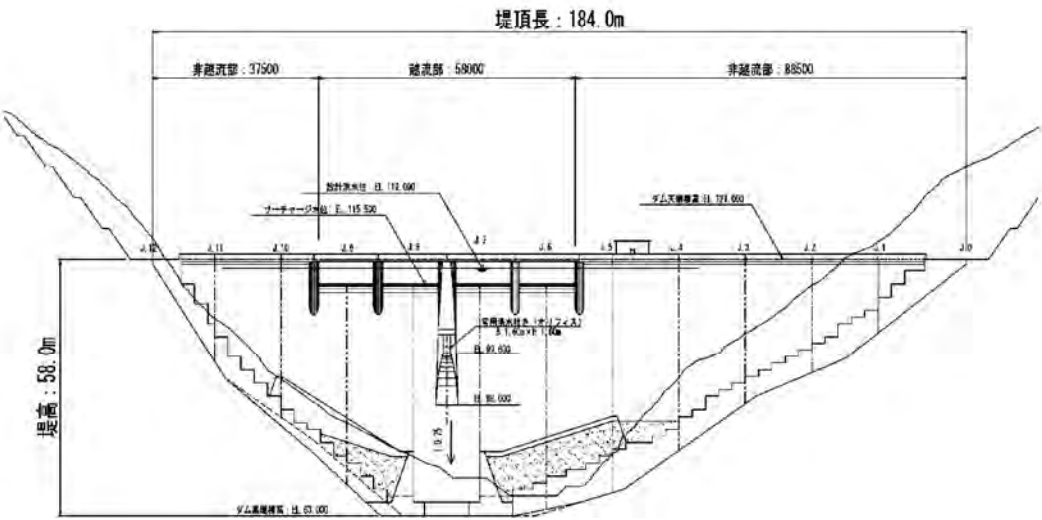
図 5.28 下流面図
