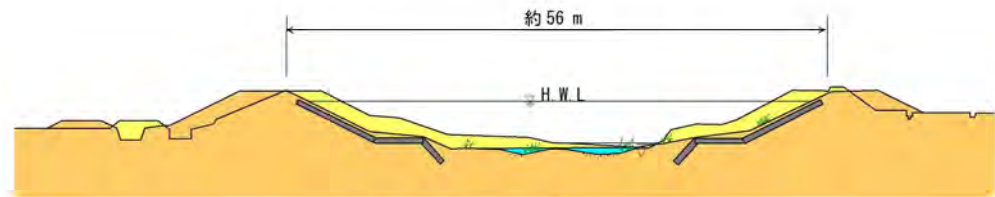
図 5.23 横断面図（イメージ）
