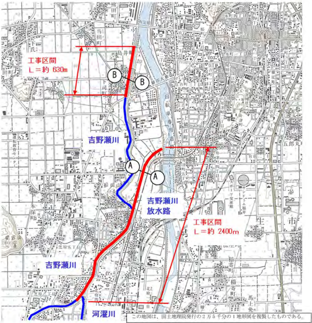
図 5.29 平面図
