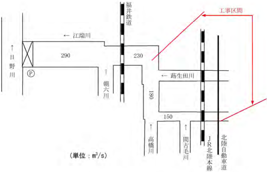
図 5.12 計画流量配分図
