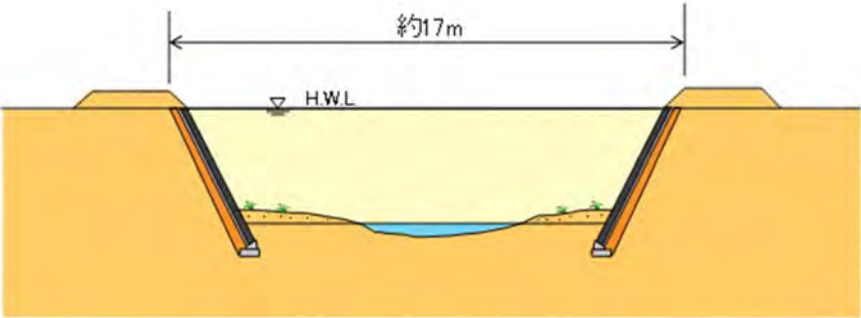
図 5.20 横断面図（イメージ）
