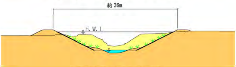
図 5.14 横断面図（イメージ）
