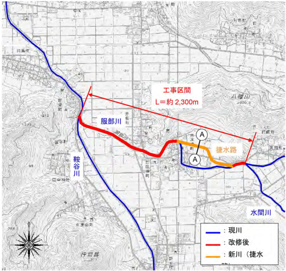
図 5.19 平面図
