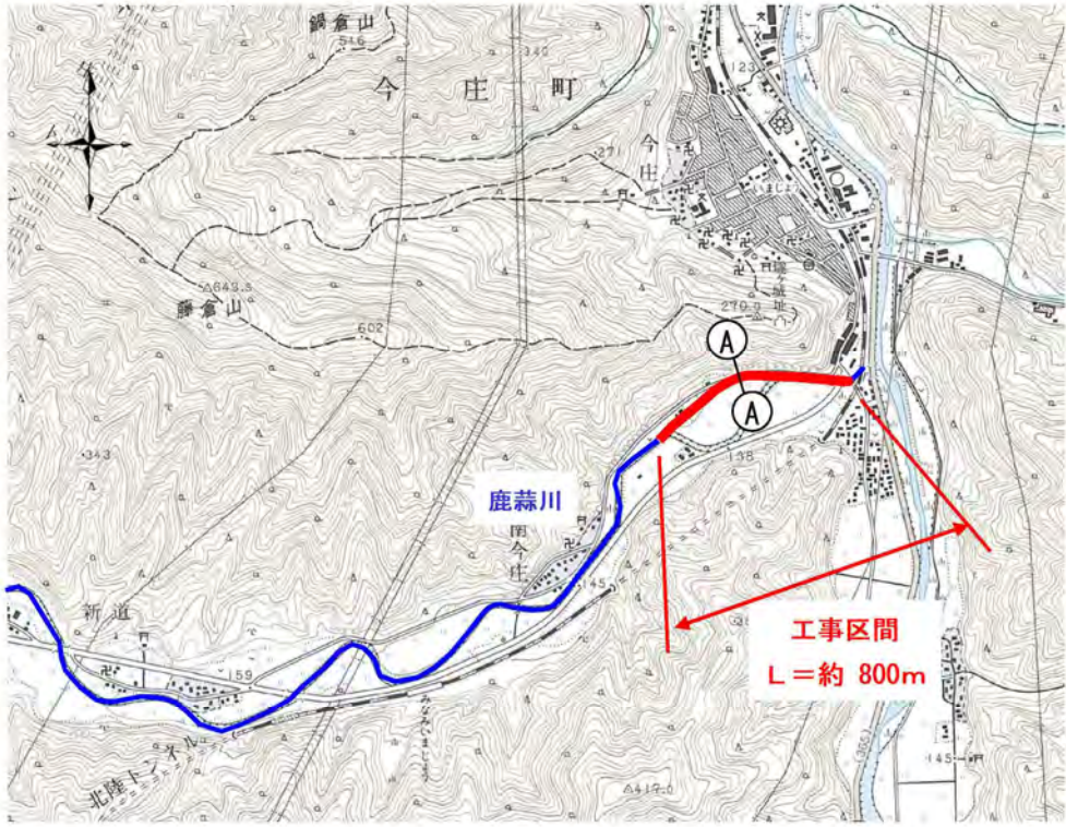
図 5.32 平面図
