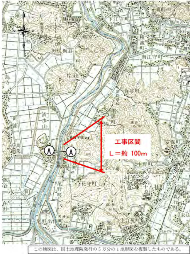
図 5.3 平面図
