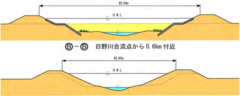
図 5.30 横断面（イメージ）
