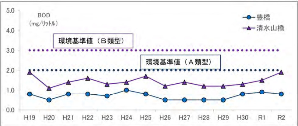
図 3.1 日野川の水質（BOD75%値）の推移
