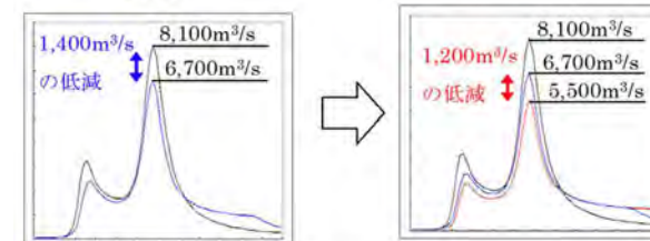
洪水調節図(中角地点)
