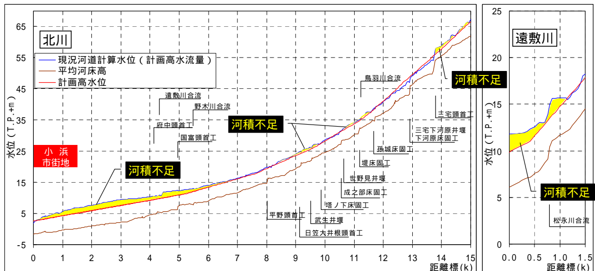
図 2.1.1 現況河道に基本方針計画高水流量が流れた場合の水位縦断図
