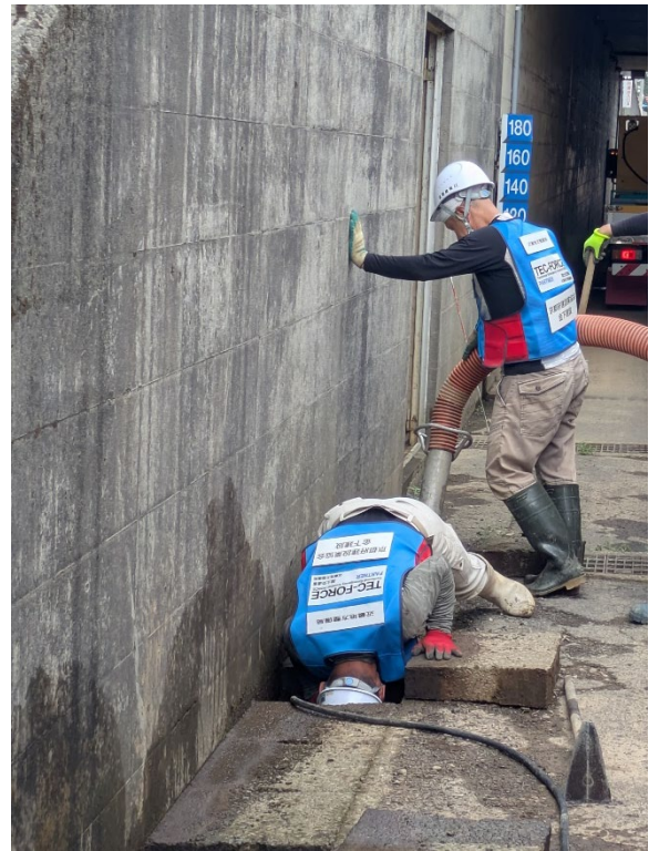
側溝内の堆積土砂に高圧噴射しながら側溝清掃車で吸引している状況
