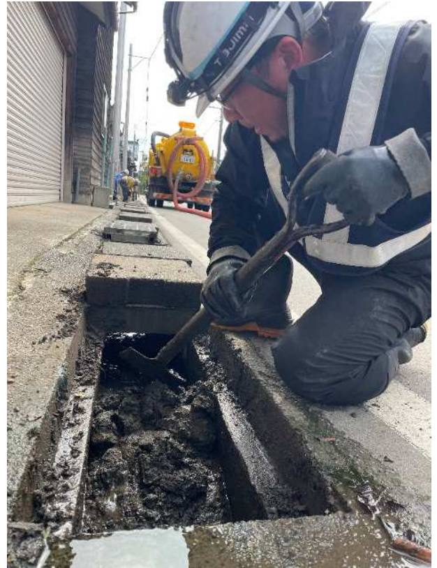
側溝内の堆積土砂を人力で撤去している状況
