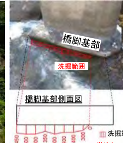
橋脚の洗掘
