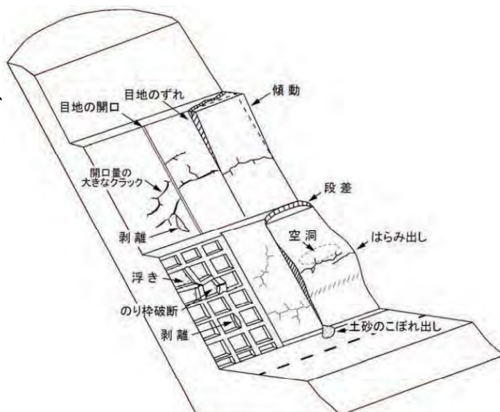
図 切土のり面の点検の着重点
