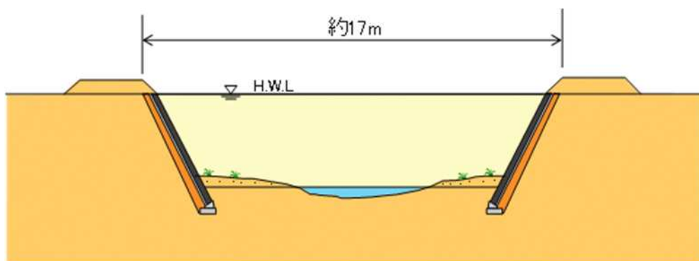
図 5.20 横断面図 (イメージ)
