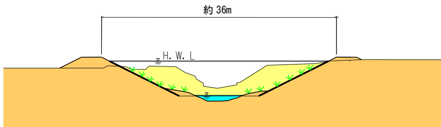
図 5.14 横断図 (イメージ)
