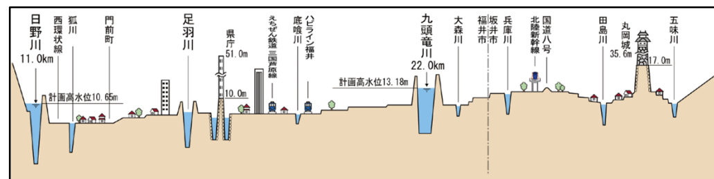
A—A' 断面
