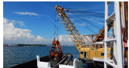
浚渫船による河道掘削の状況
