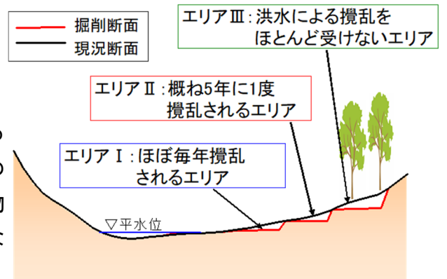
礫河原再生イメージ
