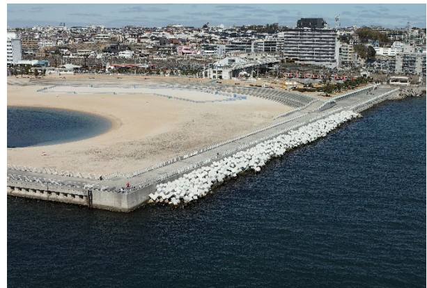
大蔵海岸消波ブロック嵩上げ(明石東部工区)
