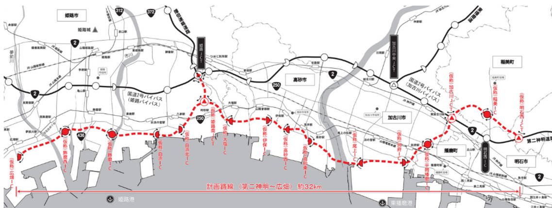
計画路線の概要図※
