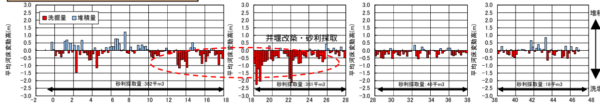
揖保川 H02～H16平均河床高変動量
