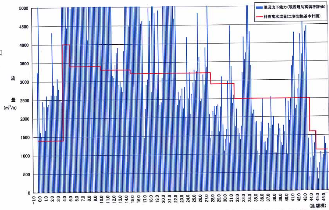
揖保川：現況流下能力図
