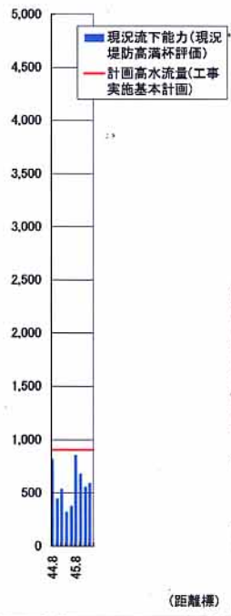
引原川：現況流下能力図
